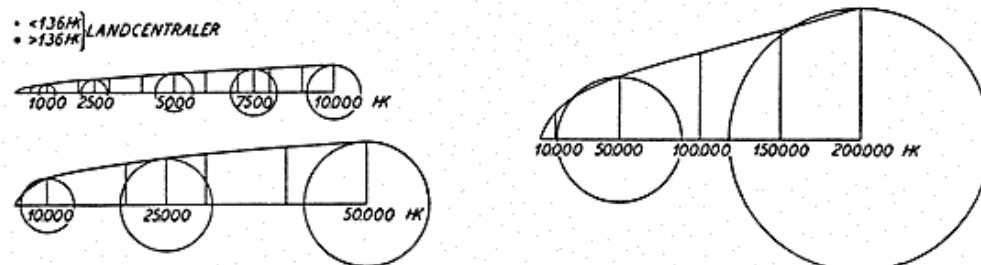
Fig. 3. Samtlige offentlige Elektricitetsværker 1911. Maskinkraft.
