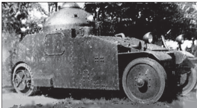
11. ábra. A páncélgépkocsi nyitott vezetőüléssel (Fotó: Éder Miklós kollekcio)
