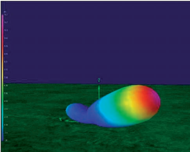
11. ábra. A földi sugárzó 3D sugárzási karakterisztikája [3]
