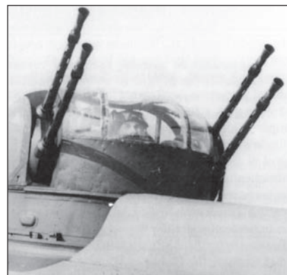
8. ábra. A Type A Mk IID torony a négy 0,303 inches (7,7 mm-es) Browning Mk II-es géppuskával
