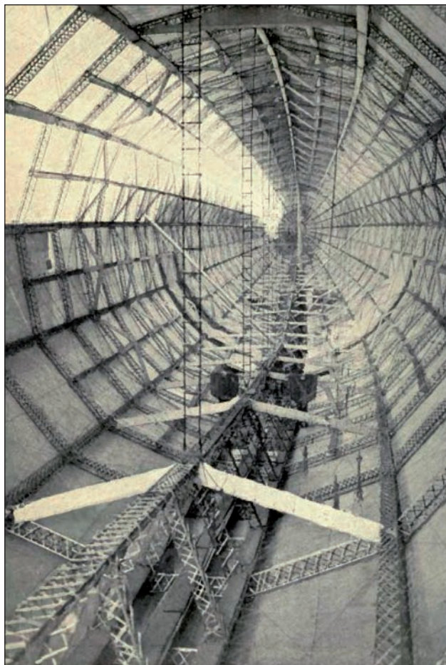
2. ábra. Az L30 (LZ-62) léghajó szerkezete belülről 1916-ban
