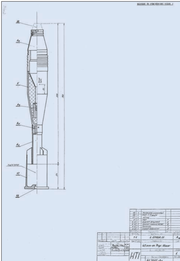
2. ábra. A 45 mm-es páncéltörő gránát rajza 1952-ből
