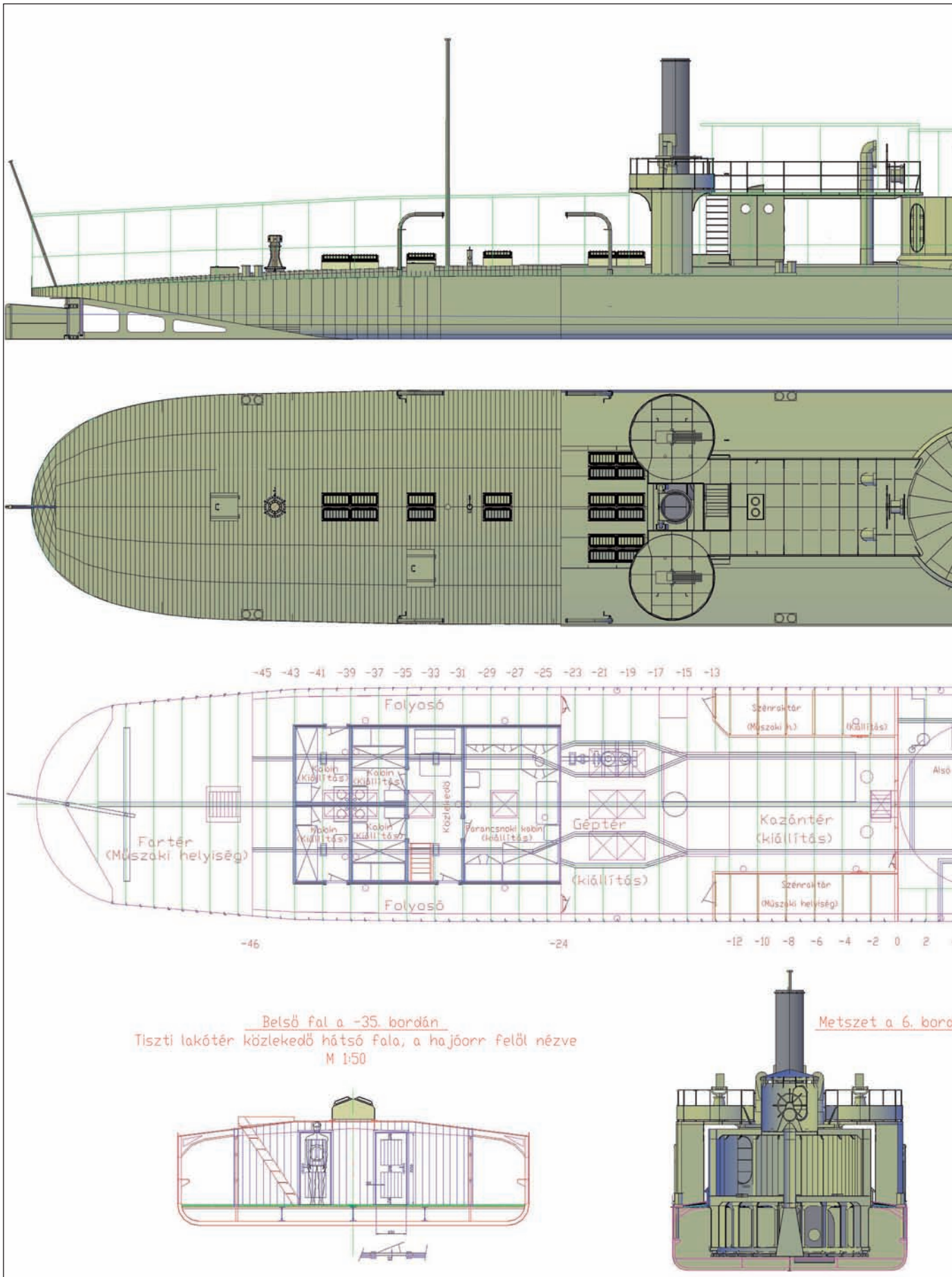
8. ábra. A LAJTA elrendezési terve. Készítette Stankovics András
