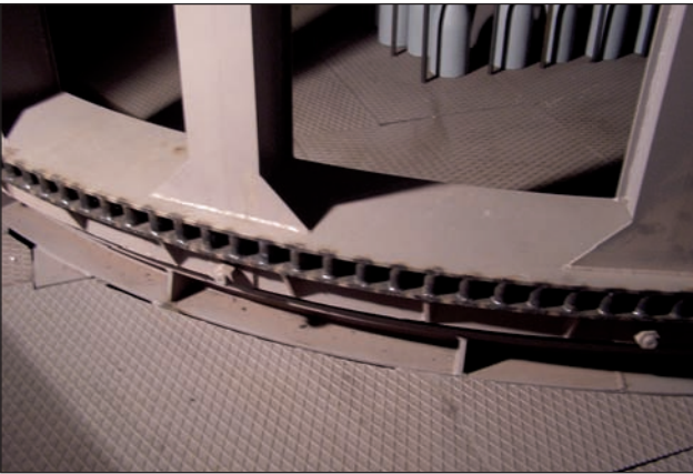
10. ábra. A torony fogasléce
