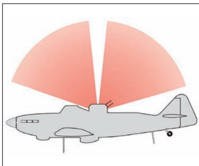
10. ábra. A Type A Mk IID torony kilövési zónája oldalról
