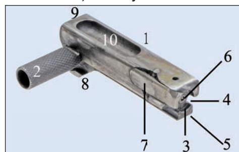
7. ábra. A rohampuska zárszerkezetének részei: 1. zártest, 2. felhúzófogantyú, 3. peremágy, 4. tölténytoló, 5. hosszanti horony (a kivető részére), 6. ütőszeg, 7. hüvelyvonó, 8. zárterelő nyúlvány, 9. reteszelőváll, 10. könnyítés
