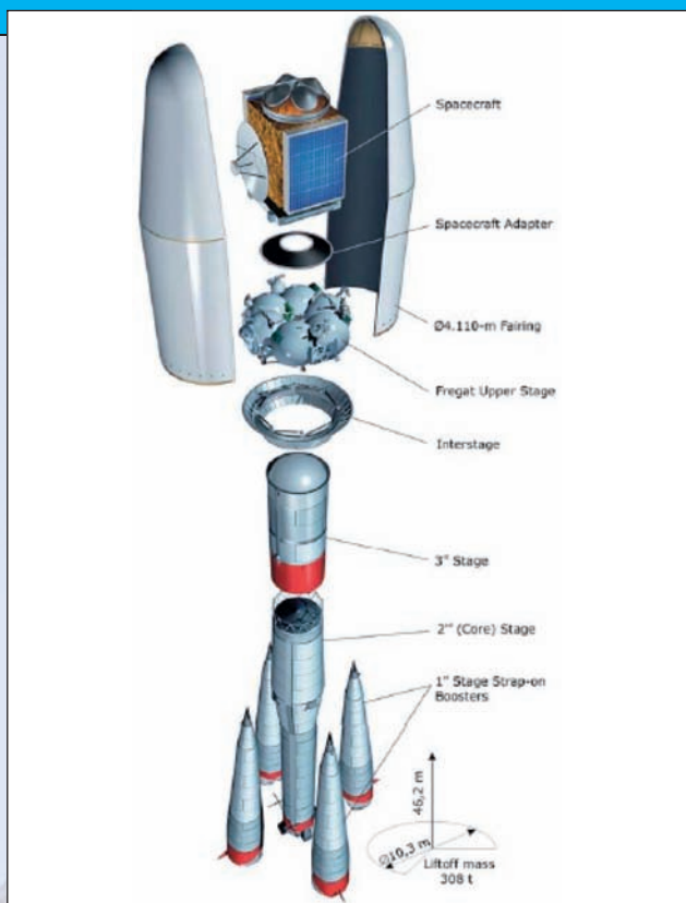
8. ábra. A kourou-i Szojuz-2 főbb részei (Soyuz Users Manual – CSG)
