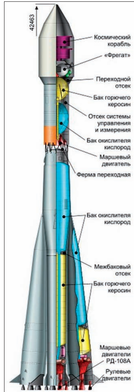
2. ábra. A Szojuz-Fregat főbb részei
