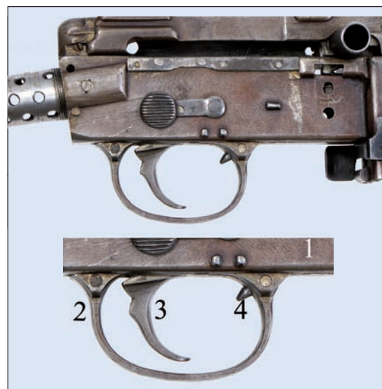
9. ábra. A fegyver sátorvasa és részei: 1. tok, 2. sátorvas, 3. elsütőbillentyű, 4. jelzőcsap
