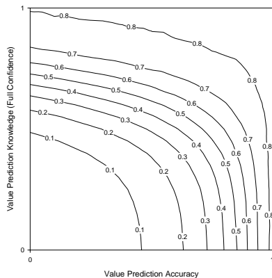
(a) Vortex
