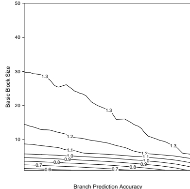
(b) Perl
