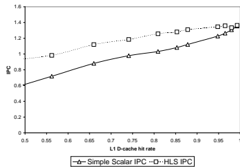
(a) Vortex
