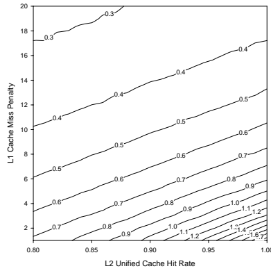
(a) Vortex
