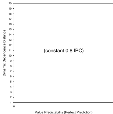
(a) Vortex
