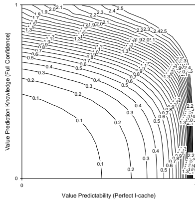
(a) Vortex
