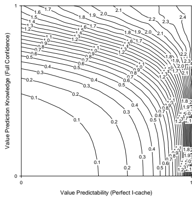
(b) Perl
