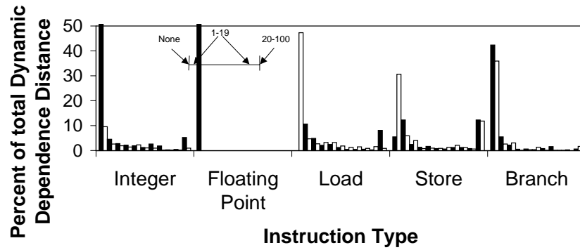
(a) Vortex
