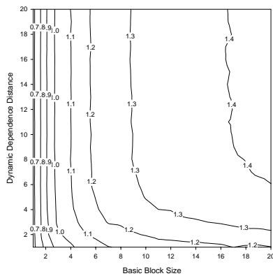
(b) Perl
