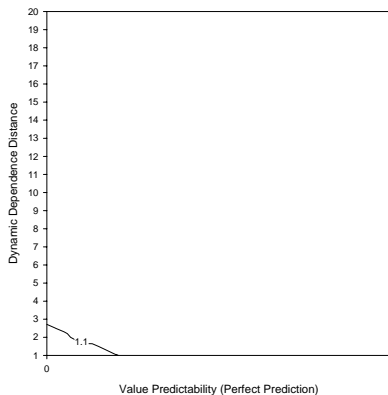
(b) Perl
