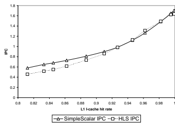
(b) Perl
