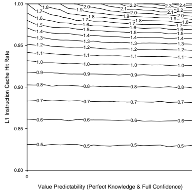
(b) Perl
