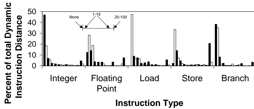
(b) Perl
