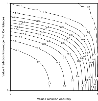
(b) Perl
