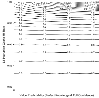
(a) Vortex
