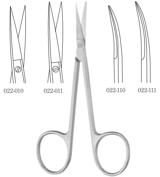
IRIS Scissors
