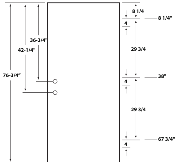
EZ-Fit Door Specs
