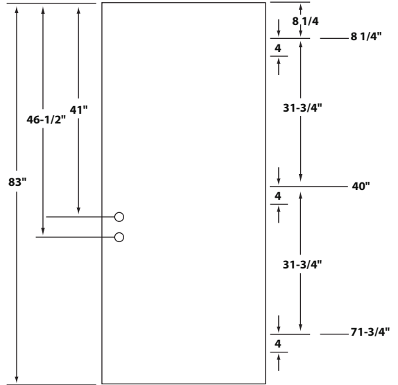
EZ-Fit Door Specs
