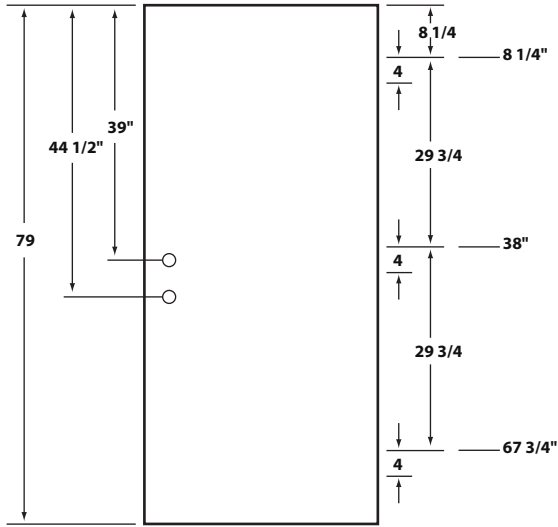
6/8 Door Specs
