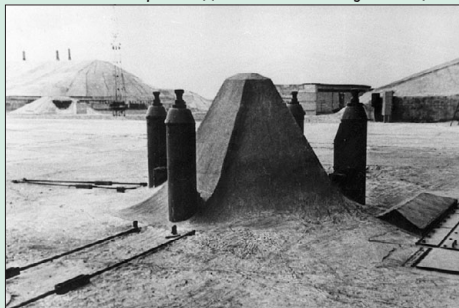
Пусковое устройство (стартовый стол) 8У255
