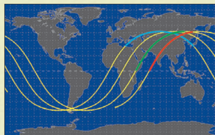
Последние витки полета ОК «Мир». Цветом выделены участки работы двигателей на торможение
