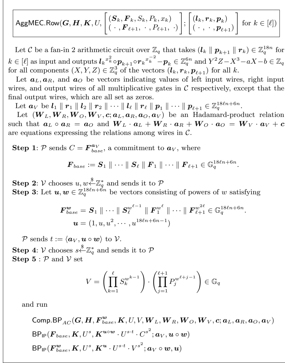
Fig. 12. AggMEC.Row
