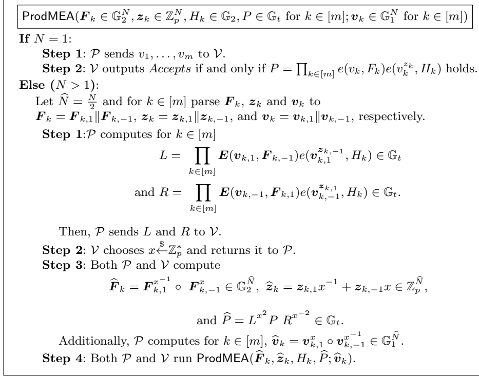
Fig. 9. ProdMEA protocol
