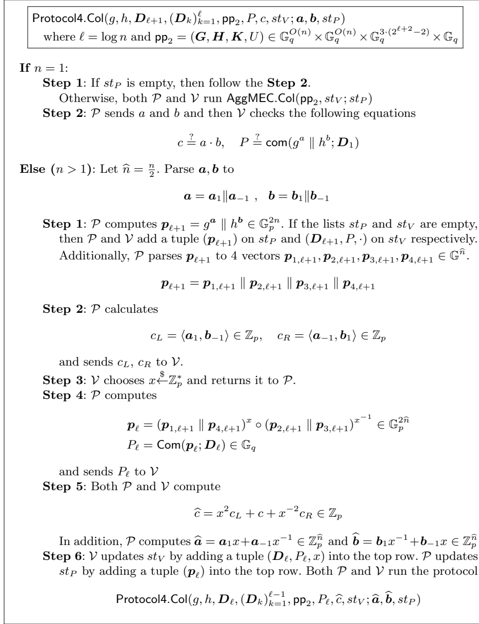
Fig. 11. Protocol4.Col
