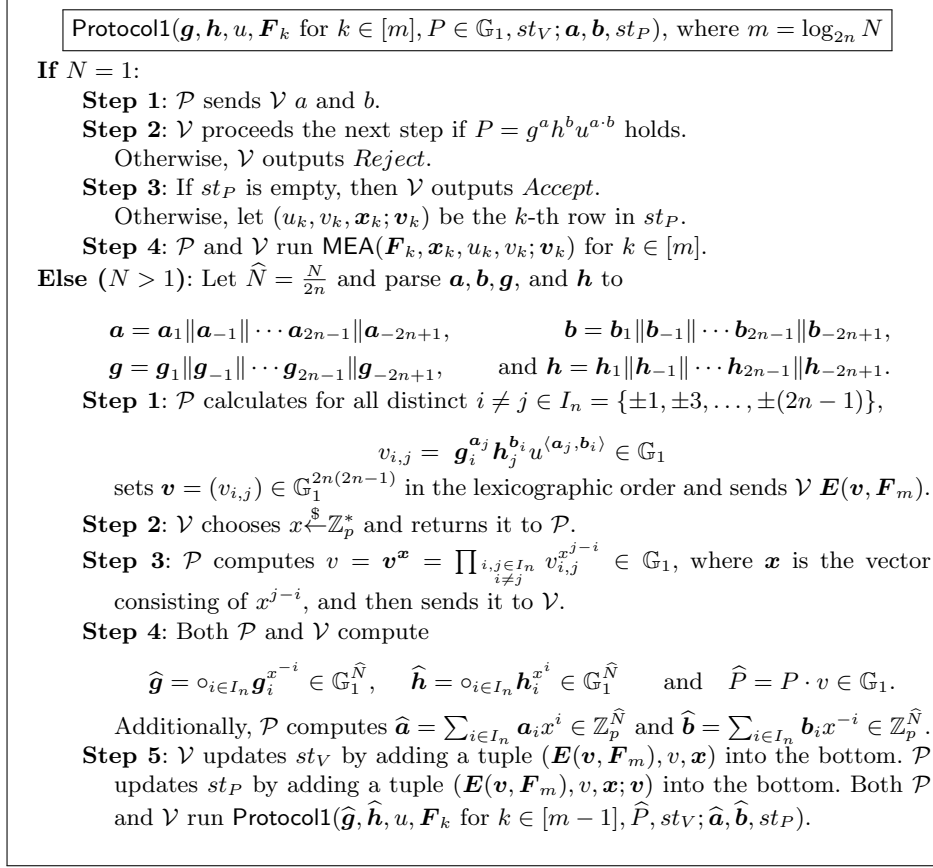
Fig. 2. Protocol1
