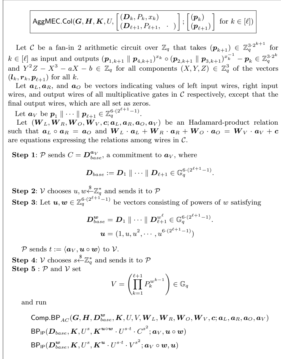
Fig. 13. AggMEC.Col
