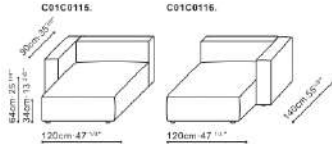
C01C0115. C01C0116. 120cm 47cm 80cm
