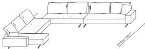
425cm 167cm C01E0505.+C01E0502.+C01E0503.-2+C01E0509.-2+C07E0511.+C01E0504.*2
