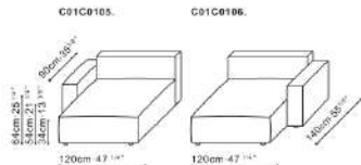
C01C0105. C01C0106. 120cm 47cm 80cm
