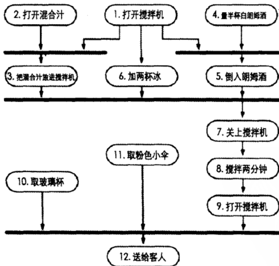
图 5.2 UML 活动图：调制冰镇果汁朗姆酒
