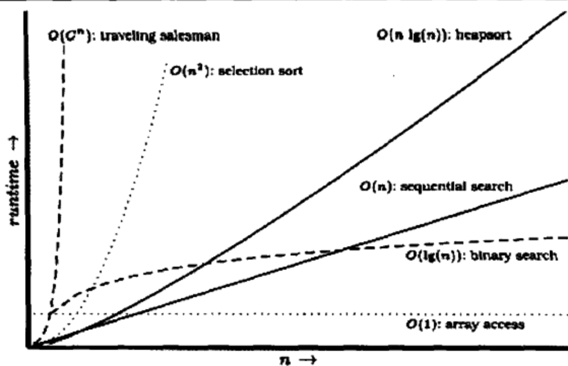
图 6.1 各种算法的运行时间
