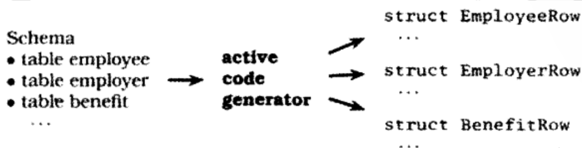
图 3.3 主动代码生成器根据数据库 schema 创建代码
