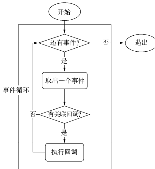
图3-11 Tick流程图
