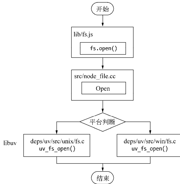
图3-12 调用示意图
