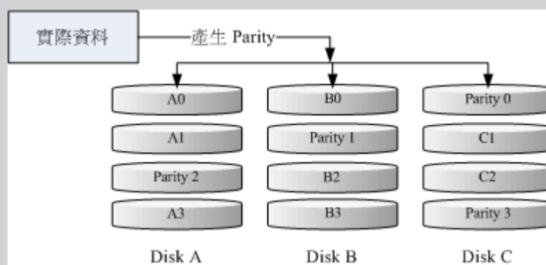
图 2.1.4、RAID-5 的磁盘写入示意图
