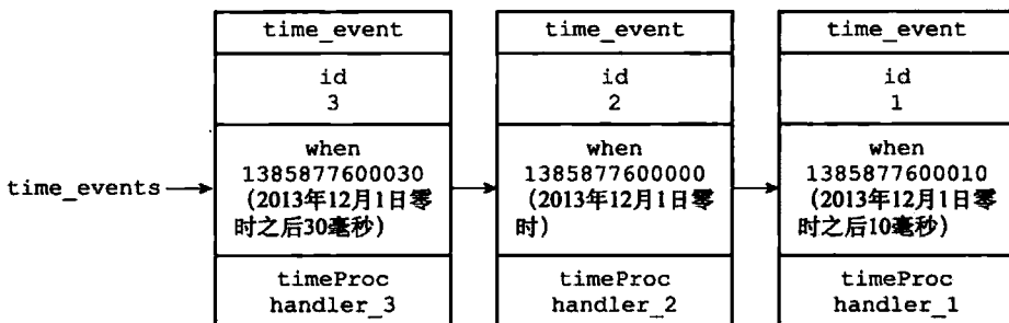
图 12-8 用链表连接起来的三个时间事件
