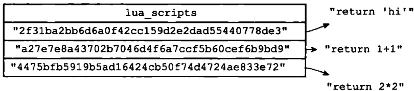
图 20-6 lua_scripts 字典
