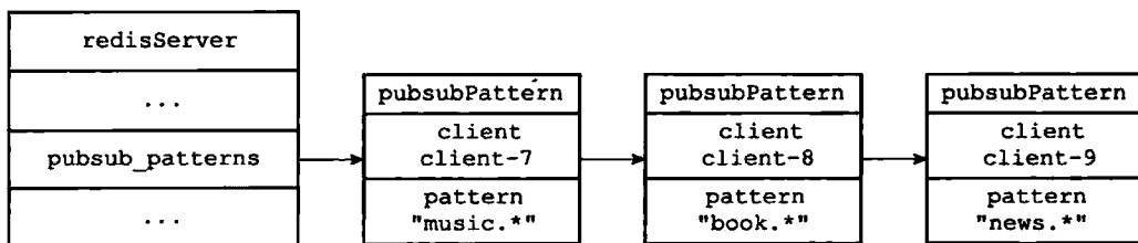
图 18-20 pubsub_patterns 链表
