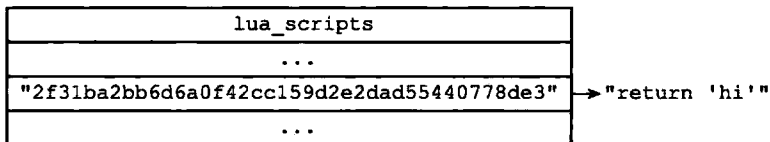
图 20-7 lua_scripts 字典
