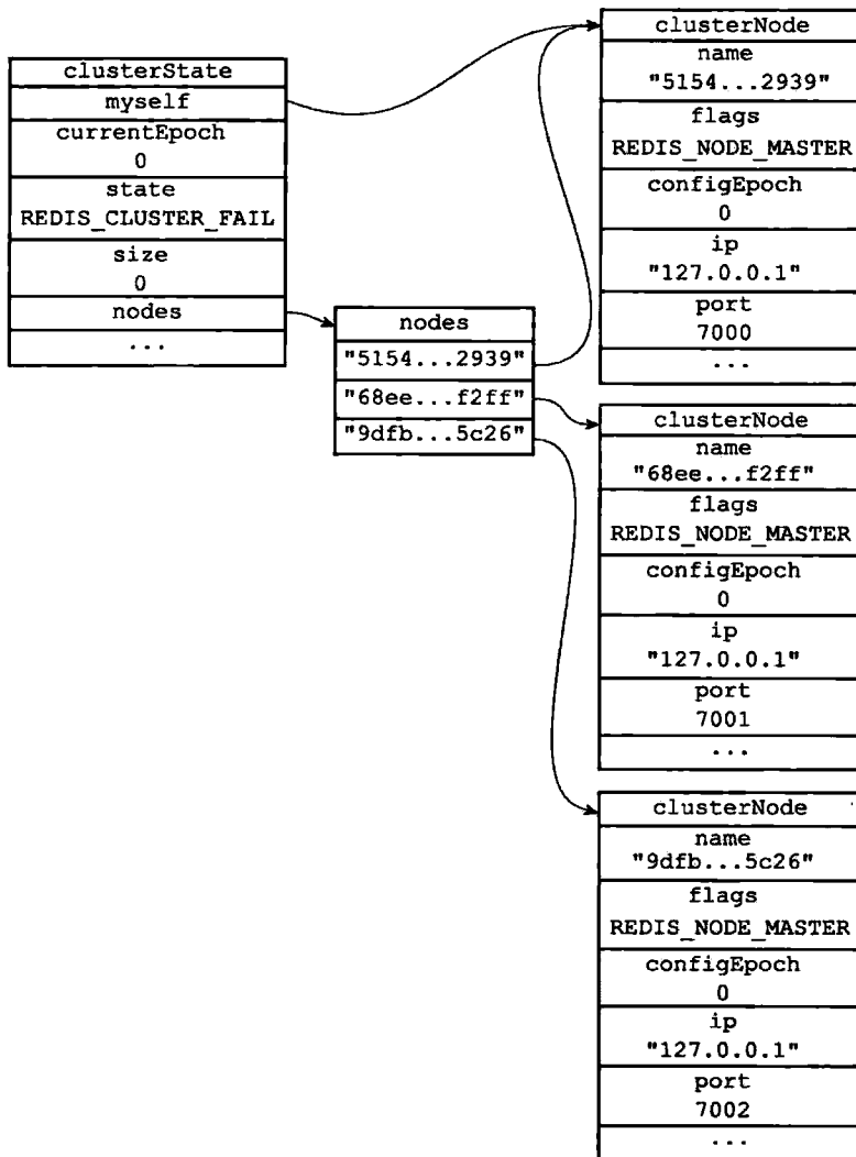
图 17-7 节点 7000 创建的 clusterState 结构
