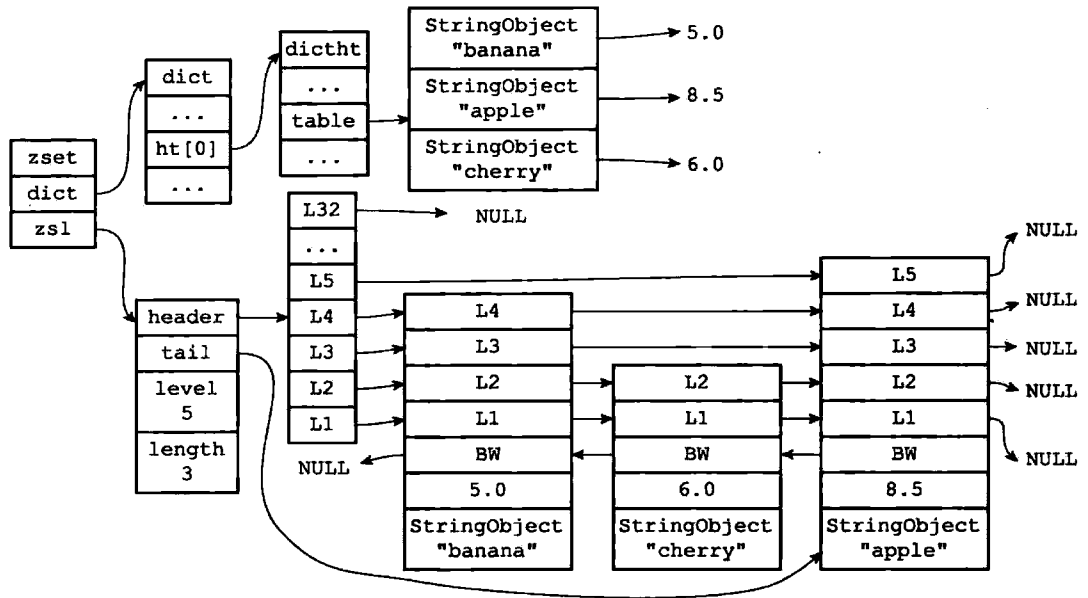
图 8-17 有序集合元素同时被保存在字典和跳跃表中
