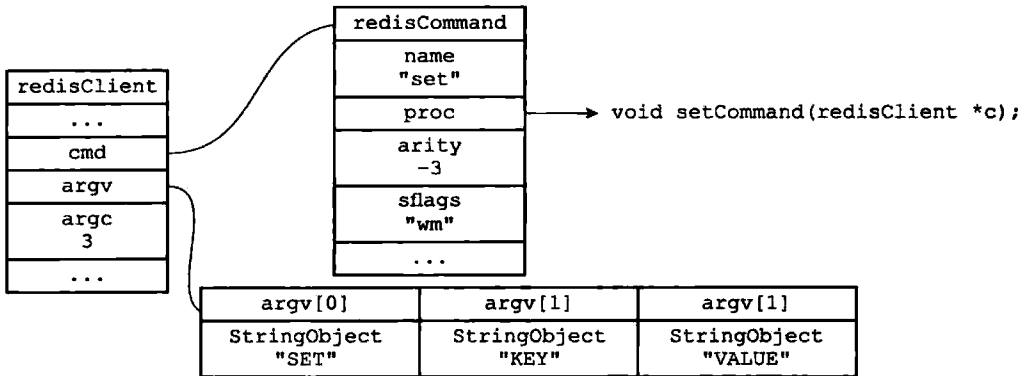
图 14-6 客户端状态
