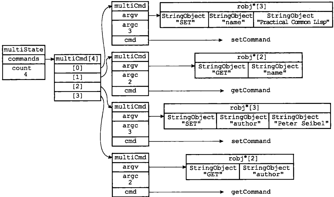
图 19-2 事务状态
