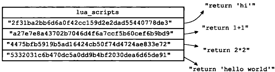
图 20-11 lua_scripts 字典
