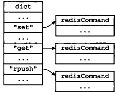
图 13-6 命令表
