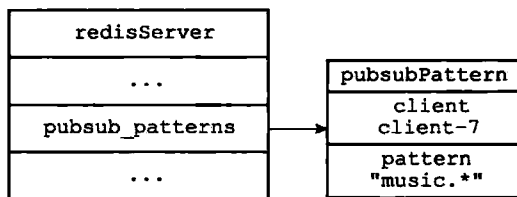
图 18-21 pubsub_patterns 链表
