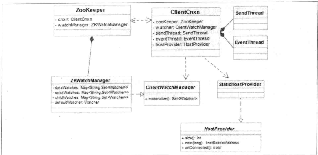
图 7-17. 客户端整体结构
