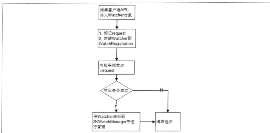
图 7-8. 客户端 Watcher 注册流程图
