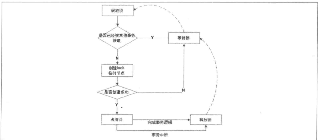
图 6-15. 排他锁的流程图
