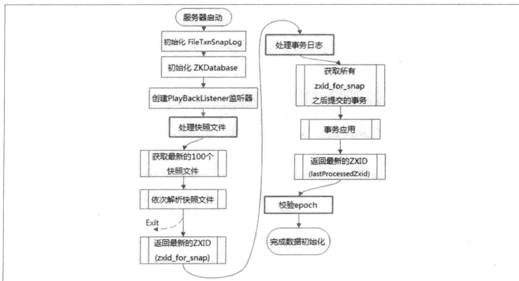
图 7-48. 服务器启动期数据初始化流程
