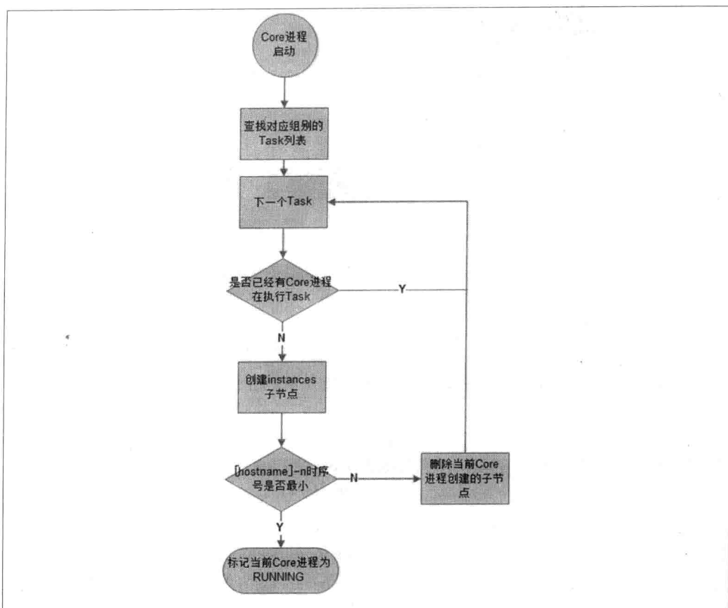
图 6-9. MySQL 数据复制组件冷备份的流程图
