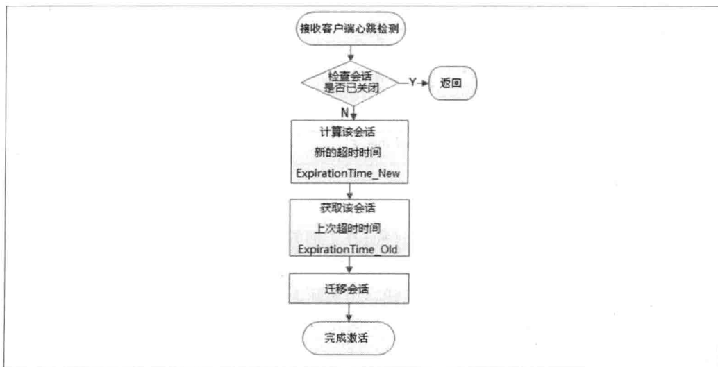
图 7-25. Leader 服务器激活客户端会话流程
