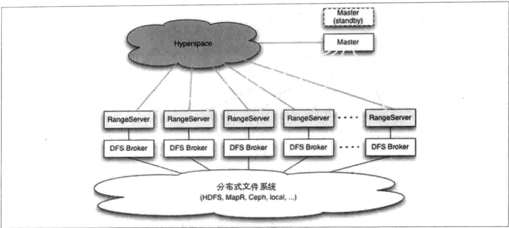
图 3-3. Hypertable 整体架构图
