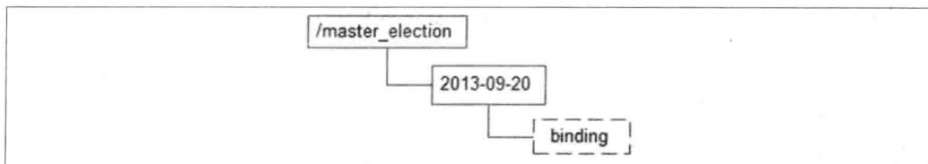
图 6-13. 一种海量数据处理与共享模型的 ZooKeeper 节点示意图
