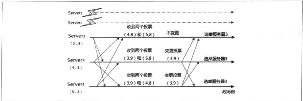
图 7-32. Leader 选举过程中发生投票变更
