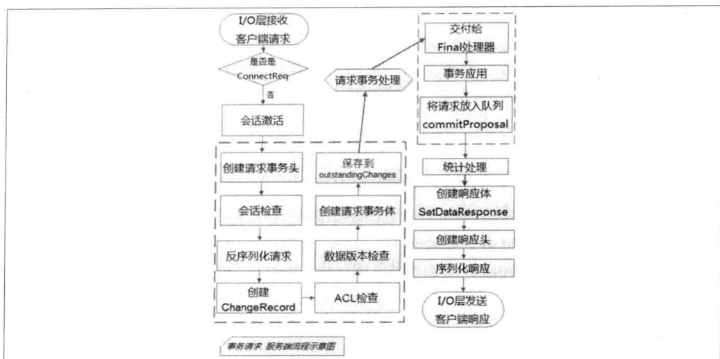
图 7-41. 事务请求处理——服务端流程示意图
