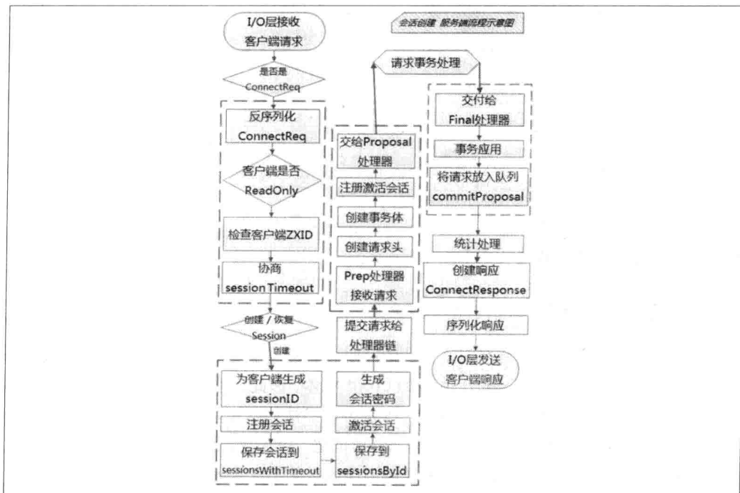
图 7-39. 会话创建处理——服务端流程示意图
