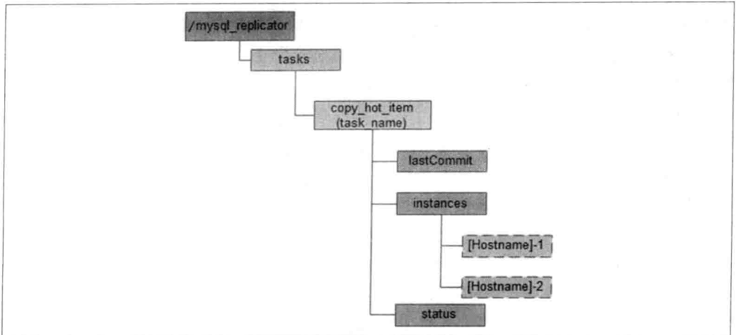
图 6-7. MySQL 数据复制组件热备份的 ZooKeeper 节点示意图
