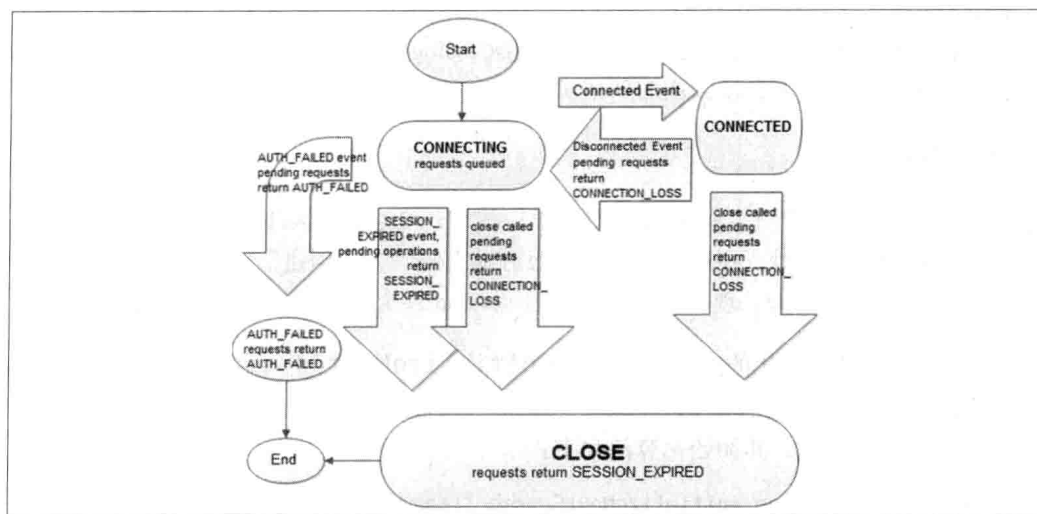
图 7-23. ZooKeeper 会话状态变更 注4
