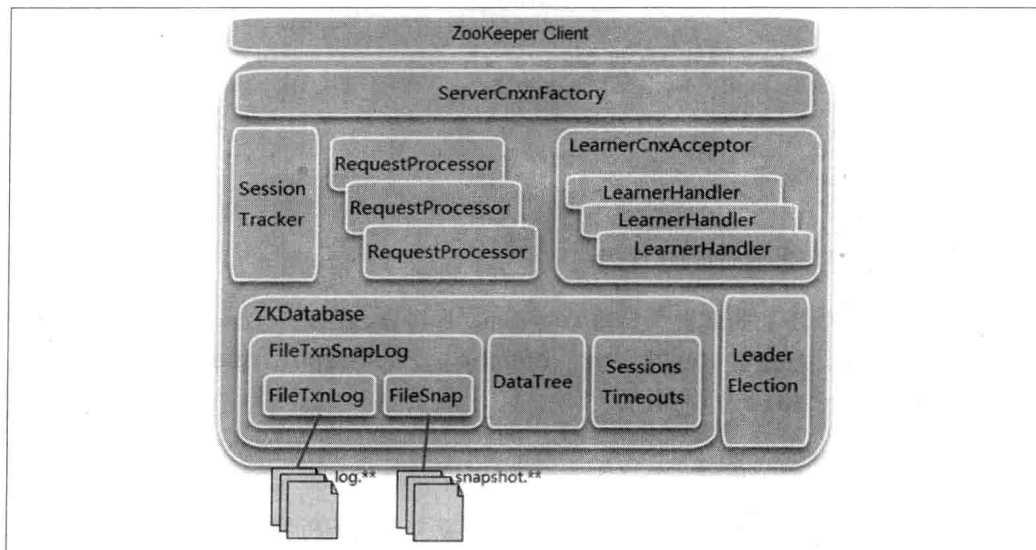
图 7-27. ZooKeeper 服务端整体架构
