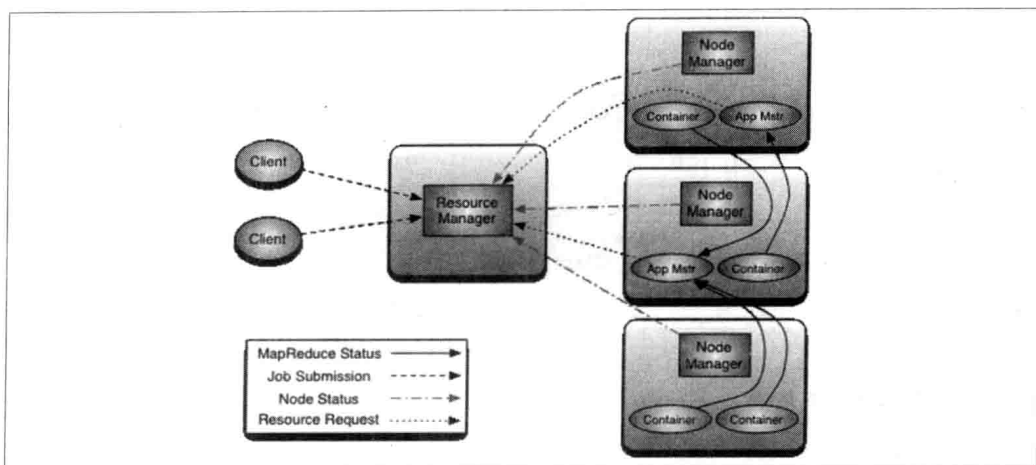
图 6-24. YARN 架构体系 注4
