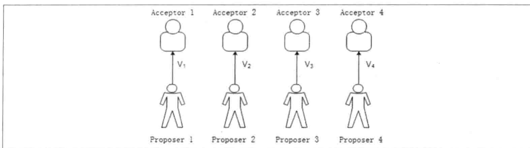
图 2-4. 不同的 Proposer 分别提出多个提案
