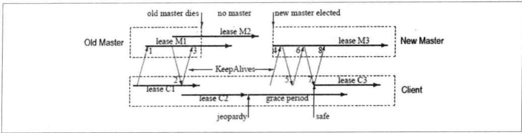
图 3-2. Chubby Master 故障恢复过程中服务端和客户端的交互示意图 注5
