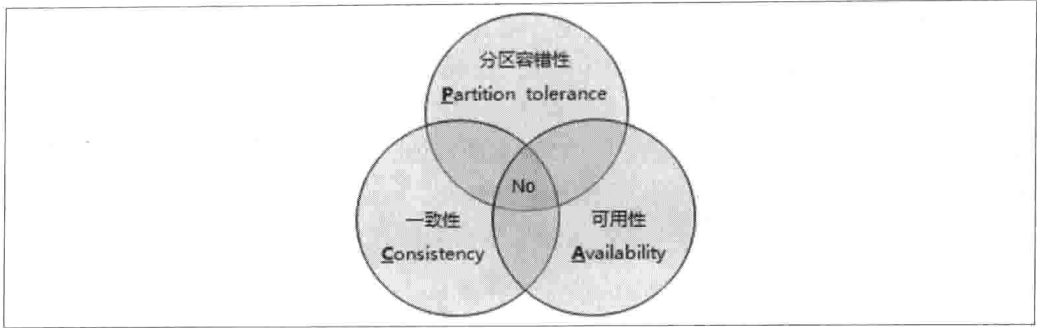
图 1-2. CAP 定理示意图
