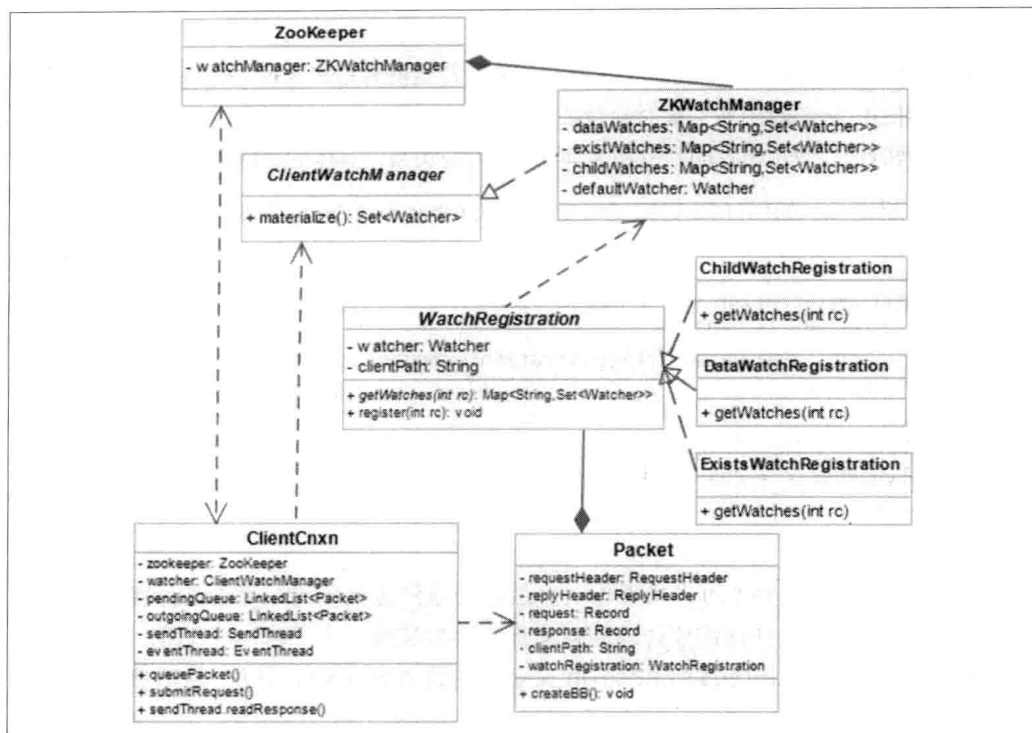
图 7-7. Watcher 相关 UML
