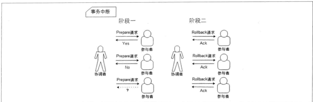
图 2-2. 二阶段提交“事务中断”示意图
