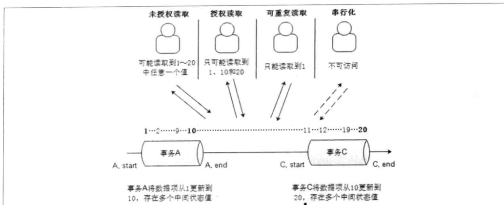
图 1-1. 4 种隔离级别示意图
