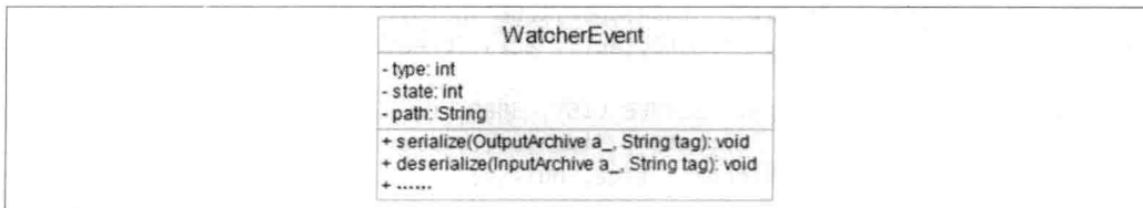
图 7-6. WatcherEvent 类图
