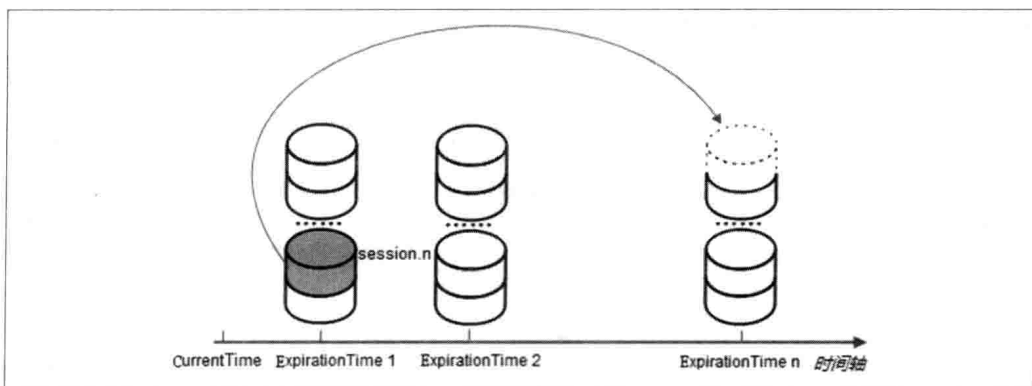
图 7-26. 会话迁移
