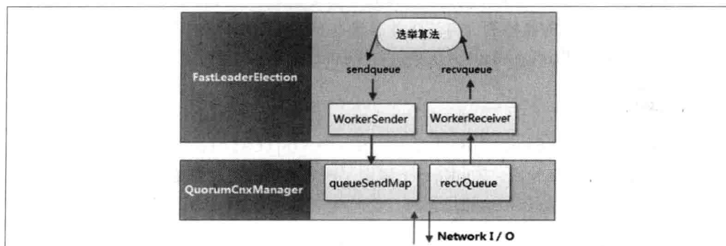
图 7-34. 选票管理
