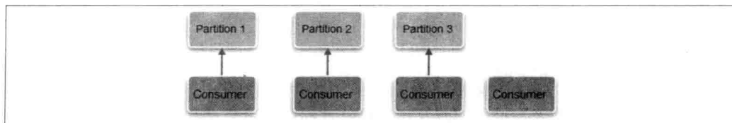
图 6-33. 消费者数大于 Topic 分区数情况下的分区消息消费示意图
