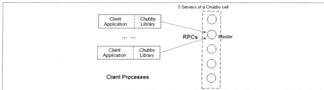
图 3-1. Chubby 服务端与客户端结构示意图
