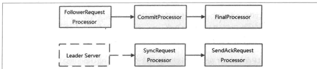
图 7-37. Follower 服务器请求处理链
