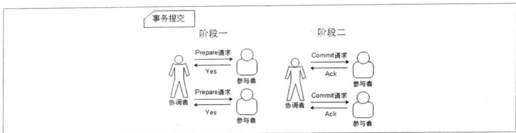
图 2-1. 二阶段提交“事务提交”示意图
