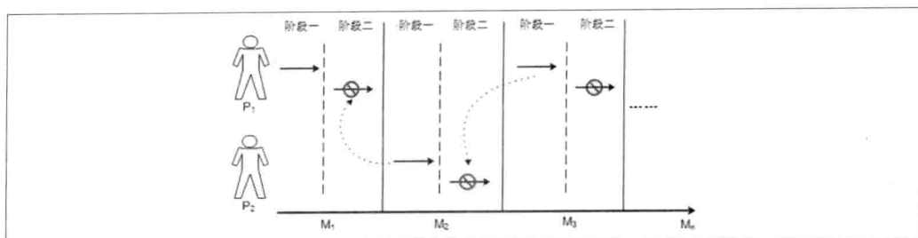
图 2-7. 两个 Proposer 分别生成提案后陷入死循环
