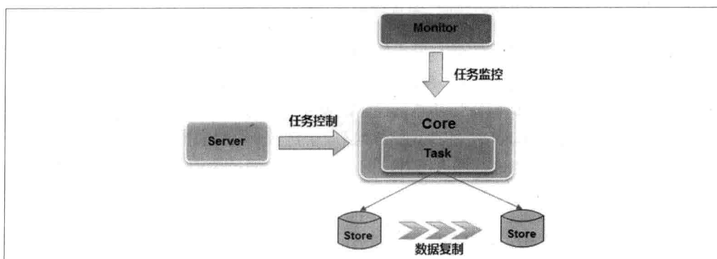
图 6-6. MySQL 数据复制子组件关系图
