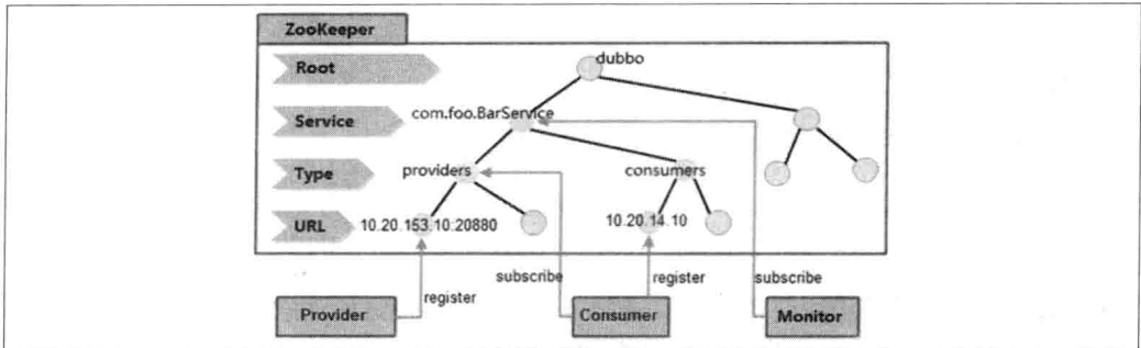
图 6-36. 基于 ZooKeeper 实现的注册中心节点结构示意图
