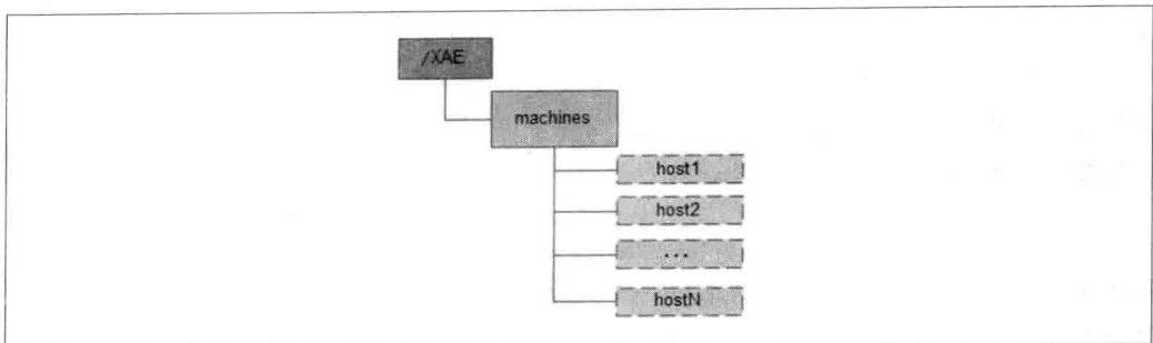
图 6-11. 在线机器列表的 ZooKeeper 节点示意图
