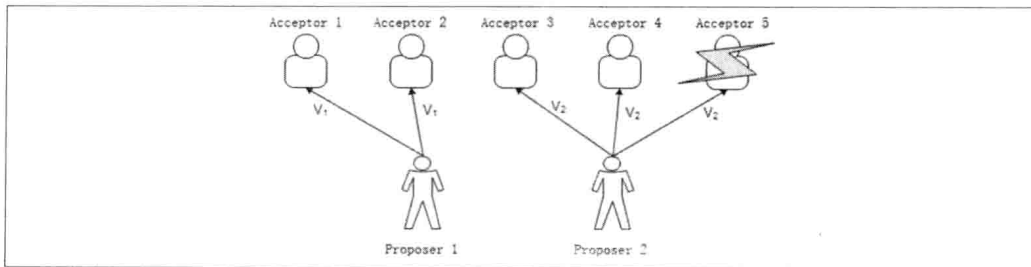
图 2-5. 任意一个 Acceptor 出现问题
