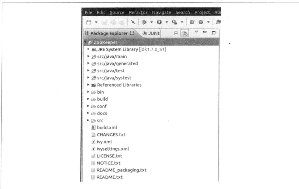
图 D-1. ZooKeeper 源代码整体结构
