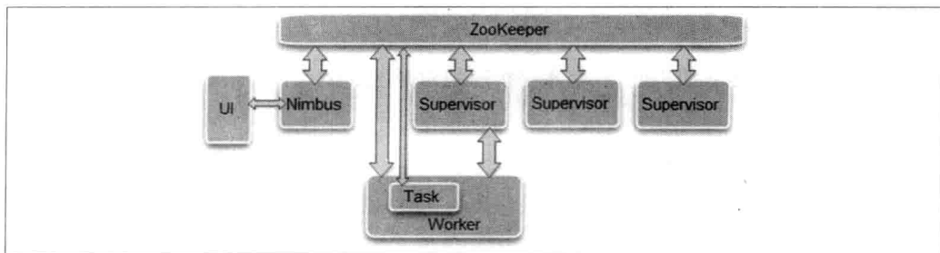
图 6-50. JStorm 整体架构图
