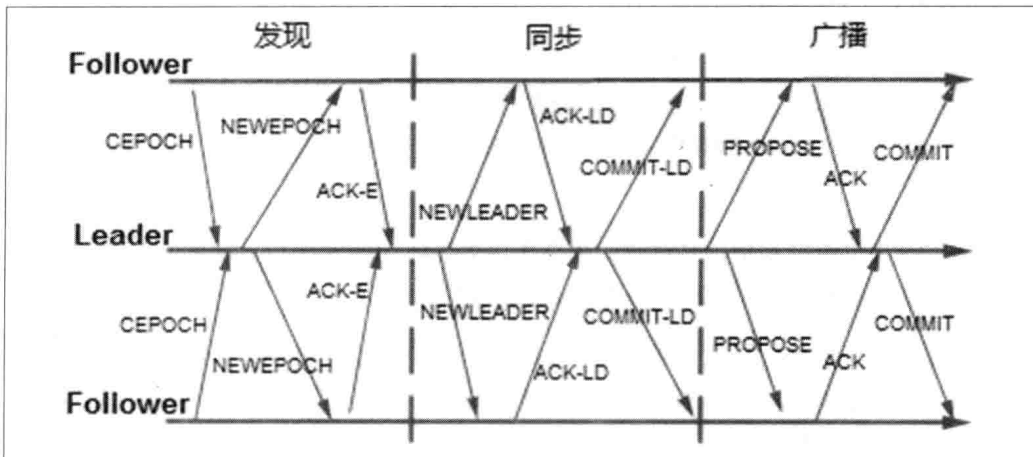
图 4-5. ZAB 协议算法描述示意图
