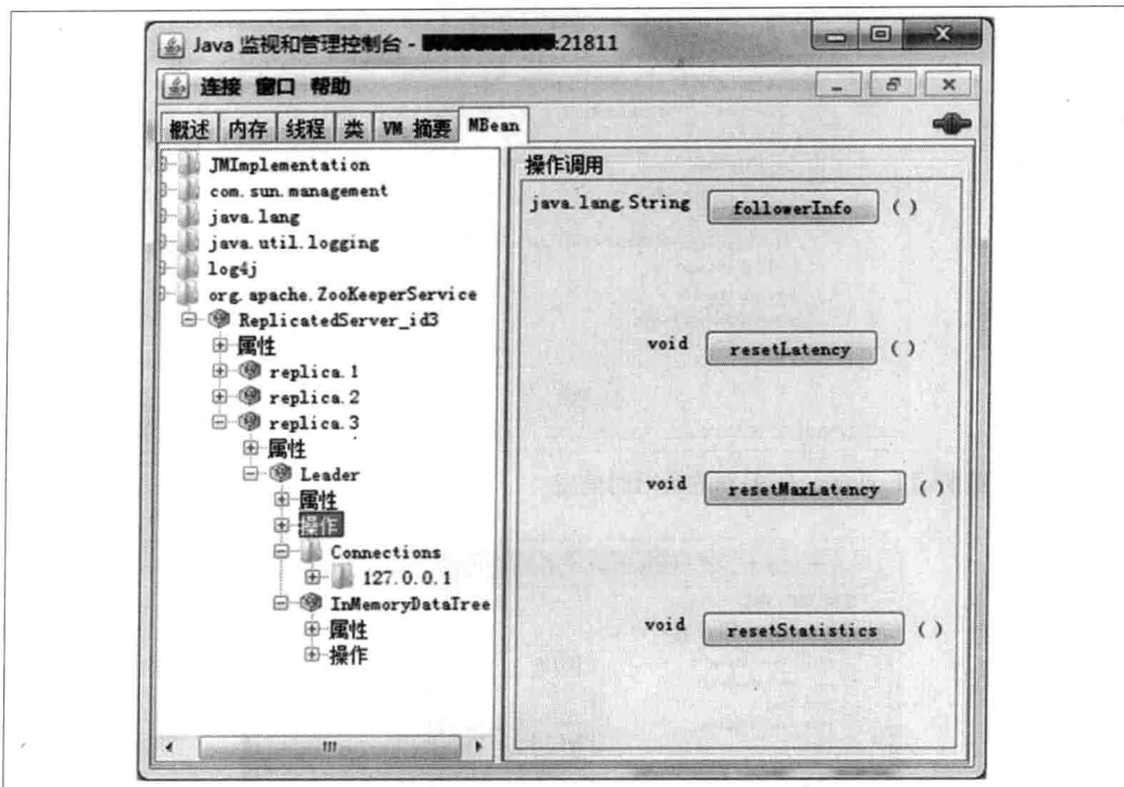
图 8-23. 查看对 Leader 服务器的操作项
