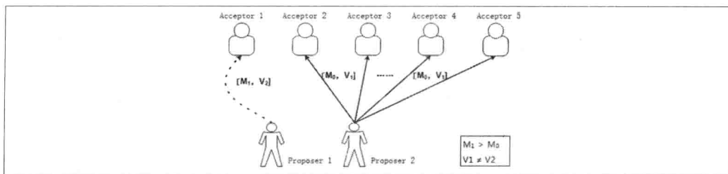
图 2-6. 一个提案可能会在某个 Acceptor 还未收到任何提案时就被选定了
