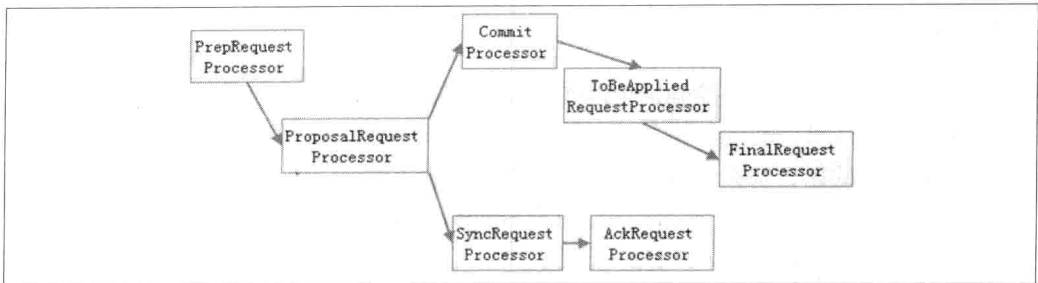
图 7-36. Leader 服务器请求处理链
