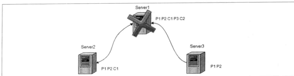
图 4-3. 崩溃恢复过程需要确保已经被 Leader 提交的 Proposal 也能够被所有的 Follower 提交
