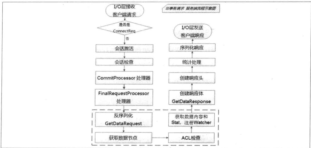
图 7-42. 非事务请求处理——服务端流程示意图
