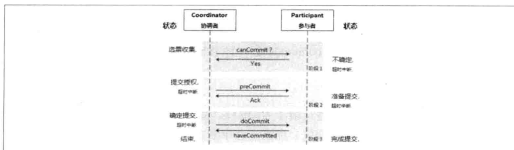
图 2-3. 三阶段提交协议流程示意图 注1
