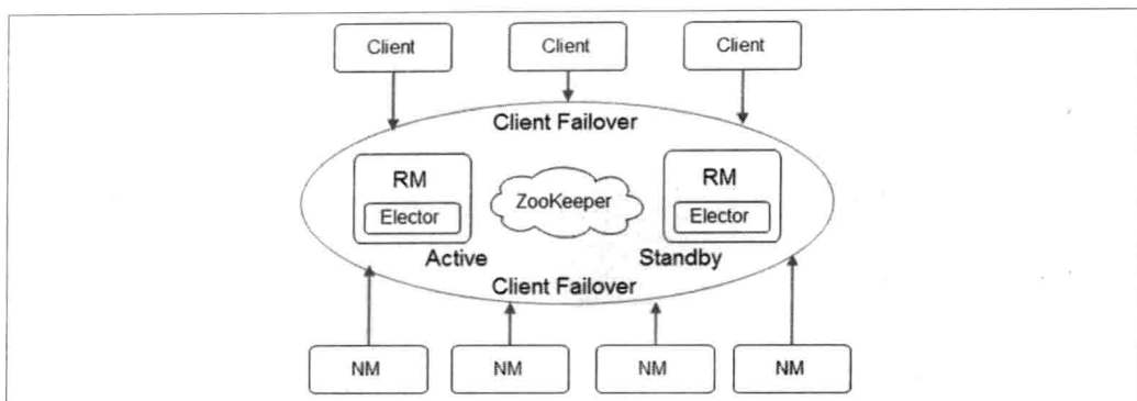
图 6-25. YARN 的 HA 架构
