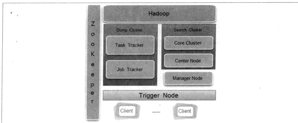
图 6-42. 终搜系统整体架构
