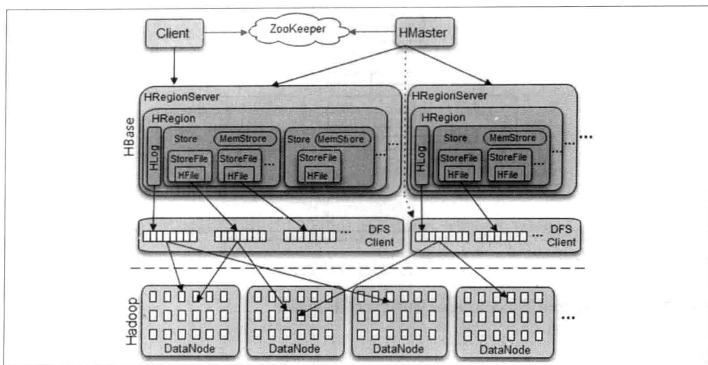
图 6-28. HBase 整体架构示意图
