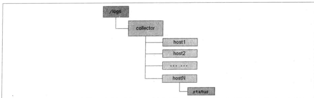
图 6-10. 分布式日志收集系统的 ZooKeeper 节点示意图
