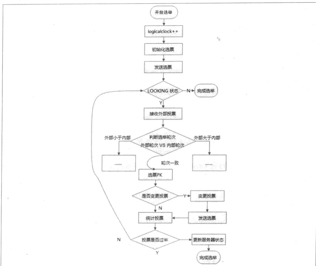
图 7-35. Leader 选举算法实现的流程示意图
