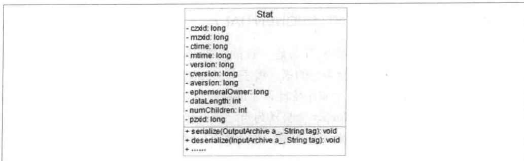
图 7-3. Stat 类图
