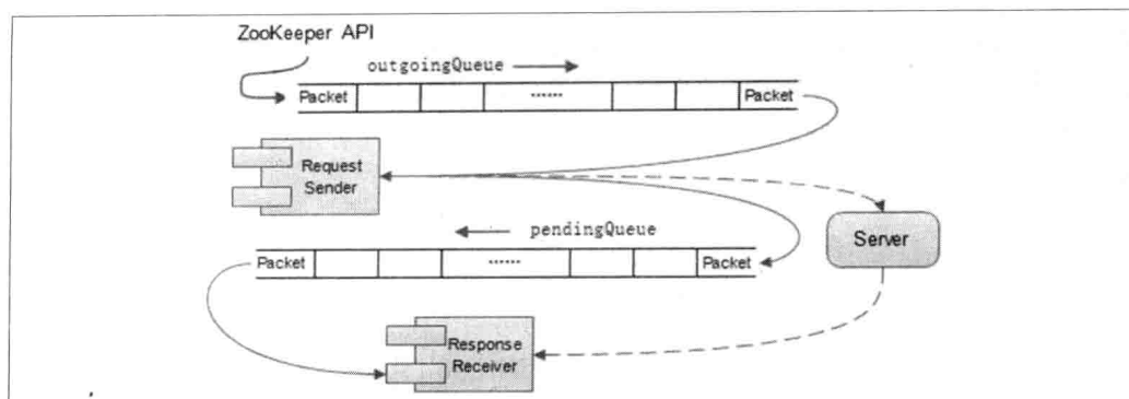
图 7-22. 请求发送与响应接收示意图
