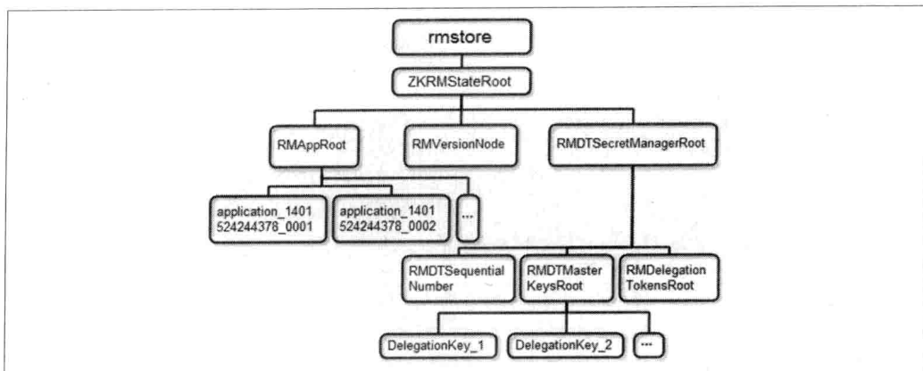
图 6-27. RMStateStore 的 ZooKeeper 数据节点结构示意图
