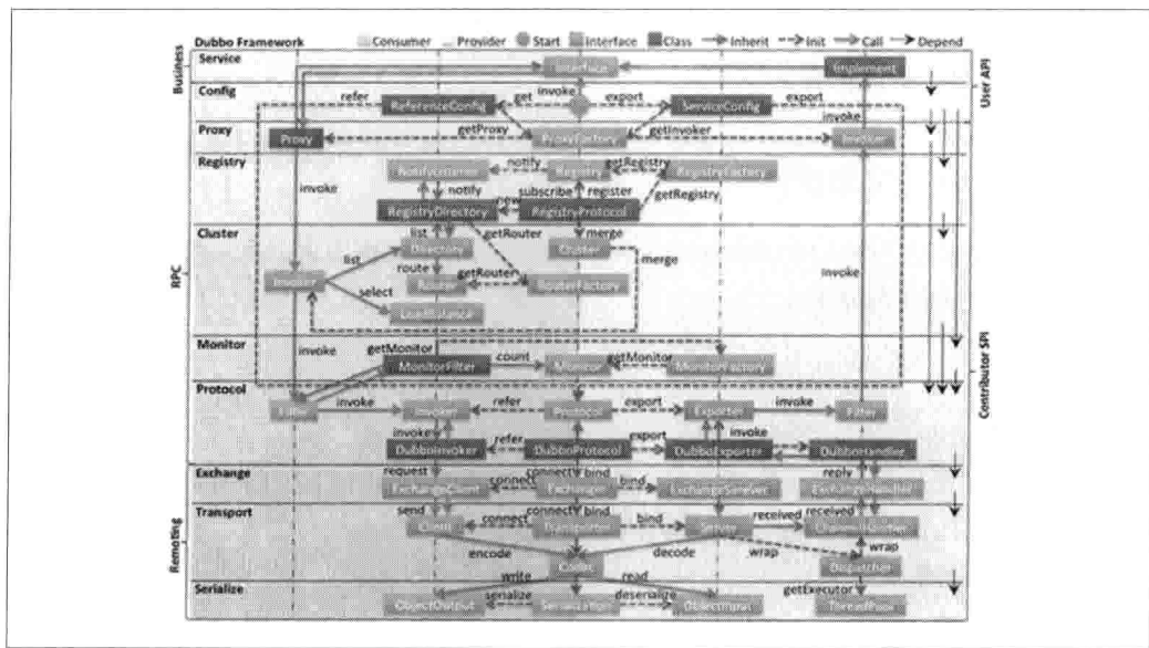
图 6-35. Dubbo 整体模块协作示意图
