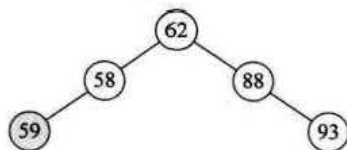
图2 不是平衡二叉树
