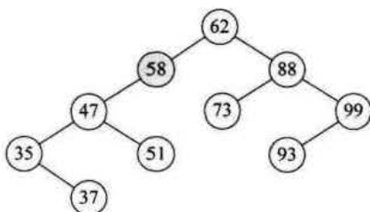
图3 不是平衡二叉树
