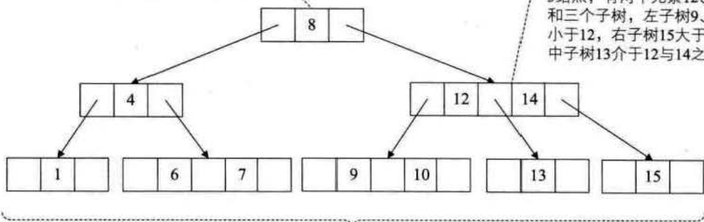
2-3树所有叶子都在同一层次
