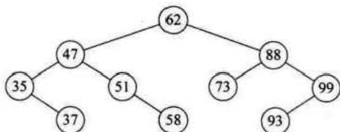
图4 平衡二叉树
