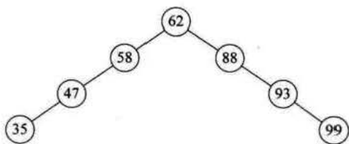
图1 平衡二叉树
