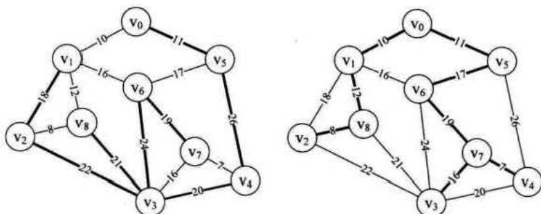
方案一 公里数=11+26+20+22+18+21+24+19=161 方案二 公里数=8+12+10+11+17+19+16+7=100
