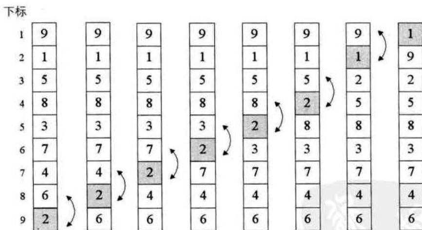
当 i=1 时将最小值 1 冒泡到顶端
