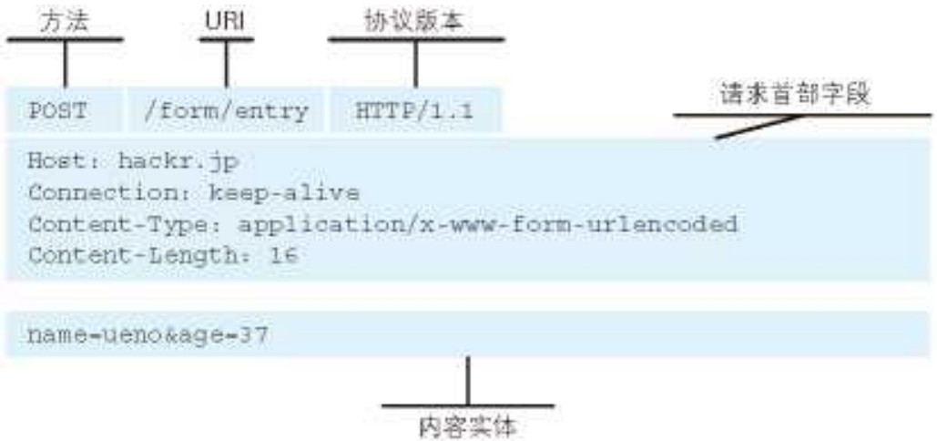
图：请求报文的构成
