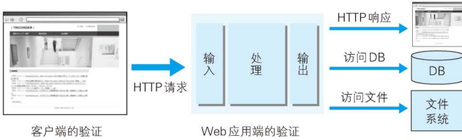
图：验证数据的几个地方
