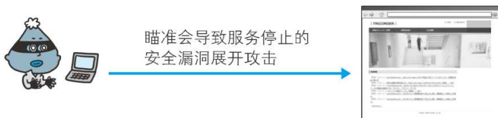
图：DoS 攻击
