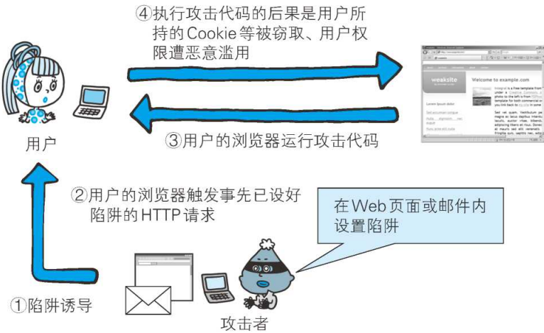
图：被动攻击
