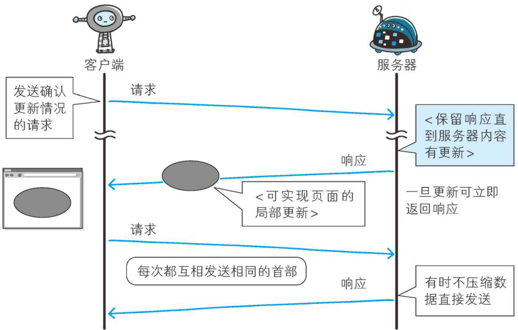
图：Comet 通信
