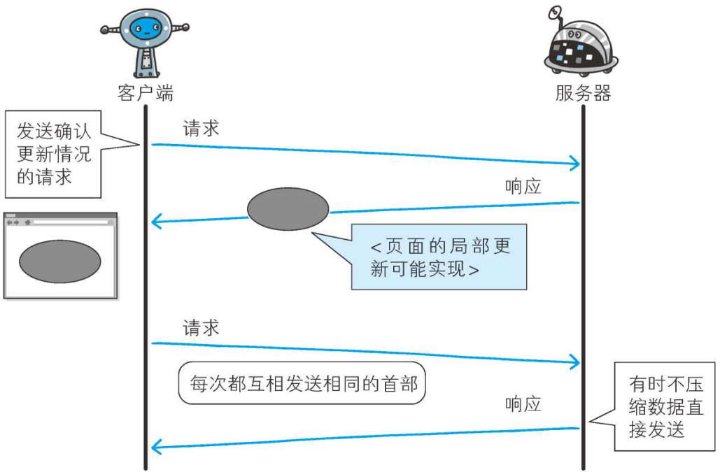
图：Ajax 通信
