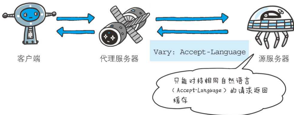
图：当代理服务器接收到带有 Vary 首部字段指定获取资源的请求时，如果使用的 Accept-Language 字段的值相同，那么就直接从缓存返回响应。反之，则需要先从源服务器端获取资源后才能作为响应返回
