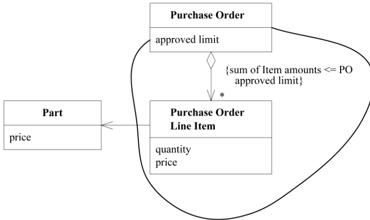
图6-11 price被复制到Line Item中，现在可以确保满足聚合的固定规则了
