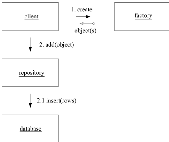
图6-23 客户使用REPOSITORY来存储新对象
