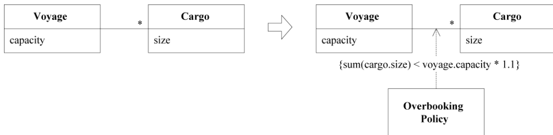
图9-11 为显式表达超订策略而重构的模型
