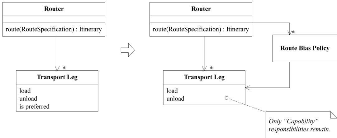
图16-7 对模型进行重构，使之符合新的分层结构
