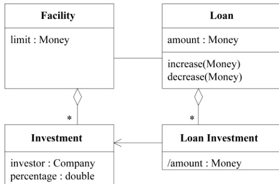
图8-1 假定放贷方股份固定的模型
