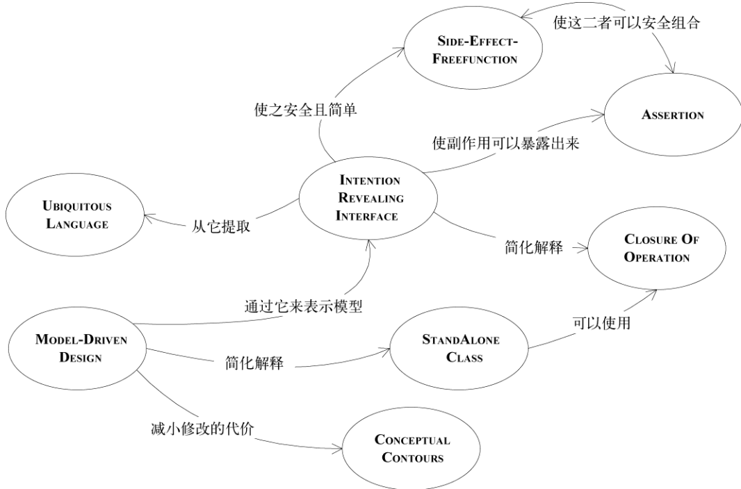
图10-1 一些有助于获得柔性设计的模式
