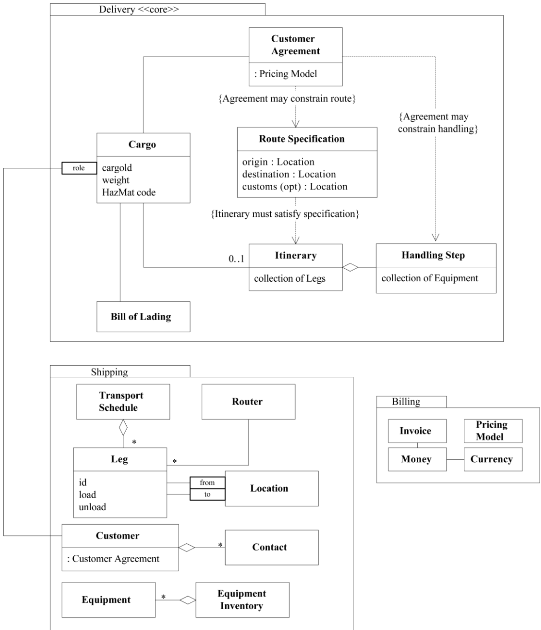
图15-3 按照客户需求可靠地运输货物是这个项目的核心目标
