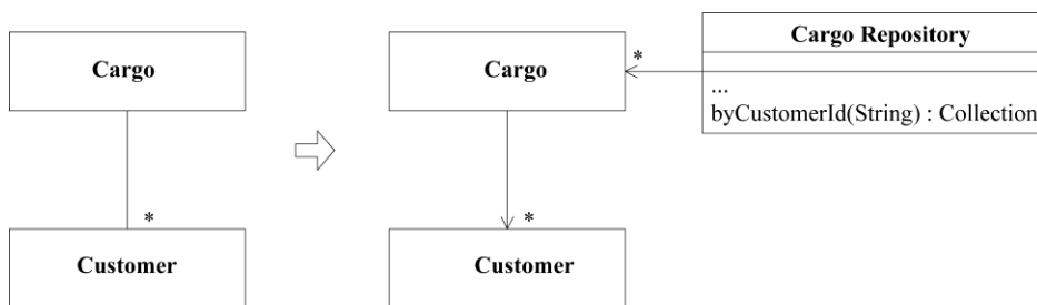
图16-5 由于双向关联会破坏分层，因此用查询来代替它
