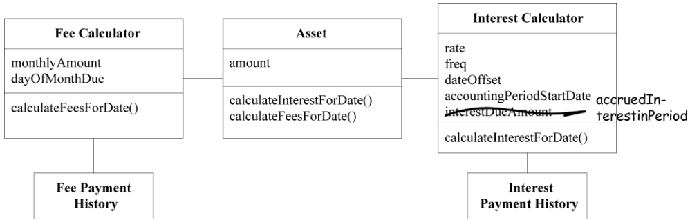
图11-5 还是原来的类图，只是把应计项目和付款分开了
