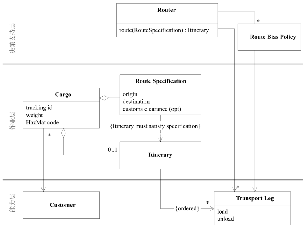
图16-8 重构后的模型
