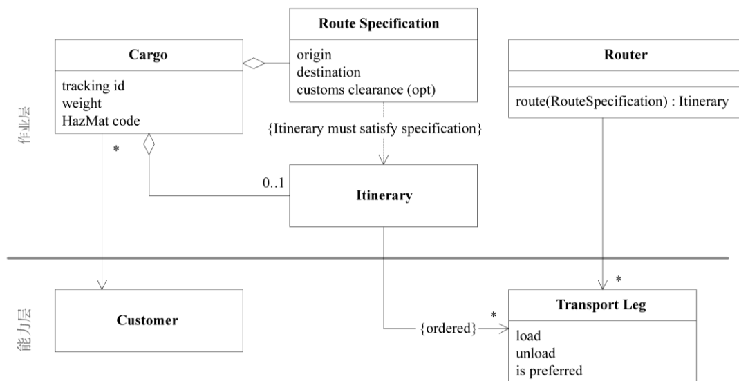
图16-6 初次对模型进行分层
