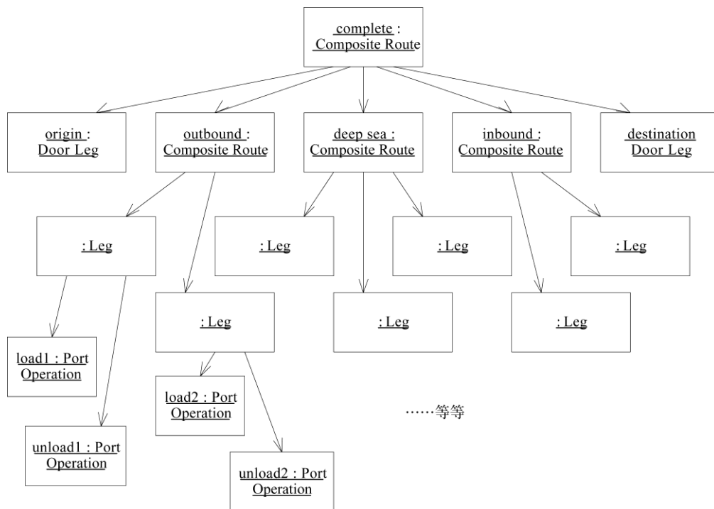
图12-9 表示了一个完整Route的实例
