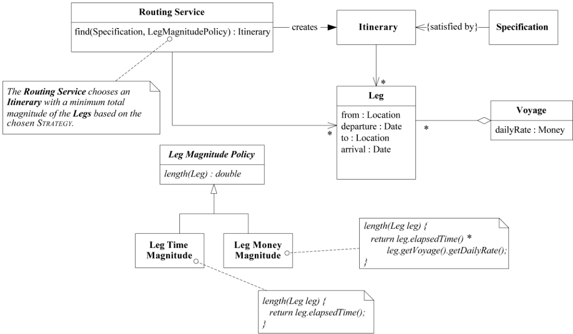
图12-2 通过STRATEGY (或者POLICY) 来确定选项 (STRATEGY是作为参数传入的)
