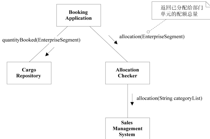
图7-10 Allocation Checker充当了一个ANTICORRUPTION LAYER，它在我们的领域模型中展现了一个到销售管理系统的可选接口
