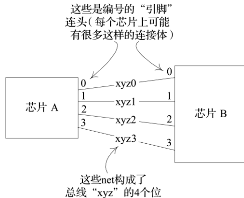
图3-2 net构成总线的示意图
