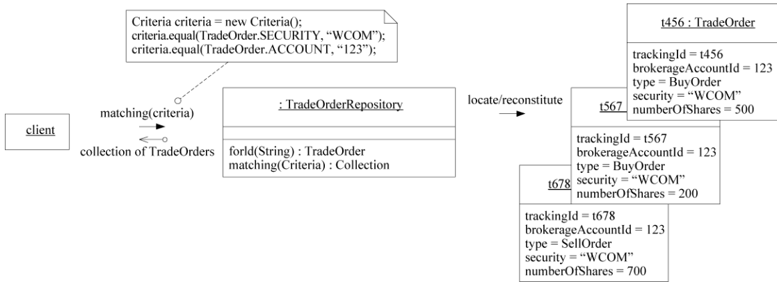
图6-20 在一个复杂的REPOSITORY中，用一种灵活的、声明式的SPECIFICATION来表述一个搜索条件
