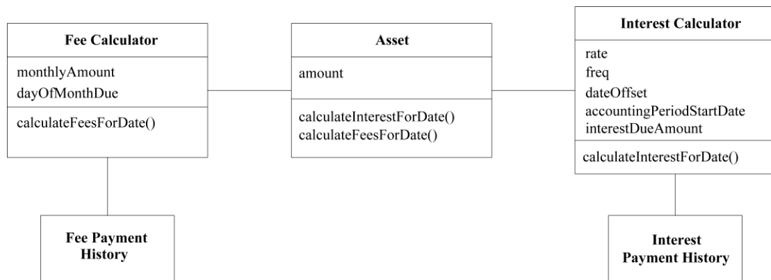
图11-1 初始的类图
