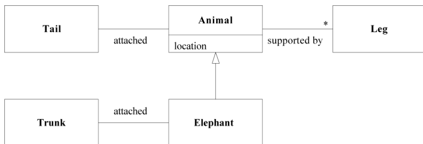
图14-12 一个更深入集成的上下文
