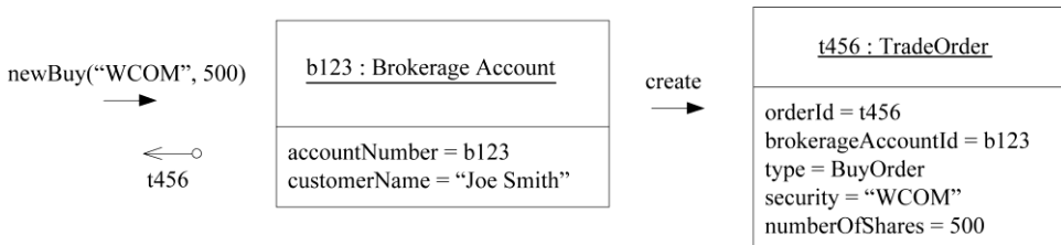
图6-14 FACTORY METHOD生成一个ENTITY，但这个ENTITY并不属于FACTORY所在的
