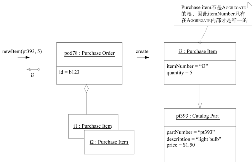
图6-13 一个FACTORY METHOD封装了AGGREGATE的扩展
