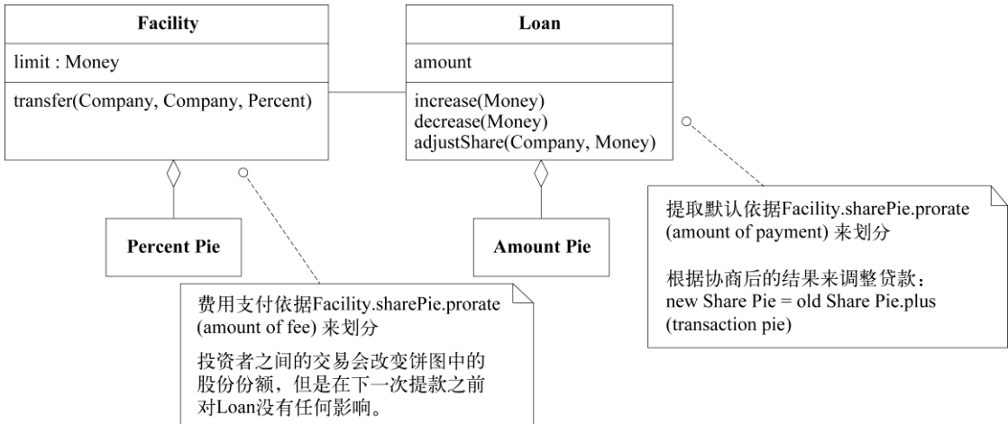
图8-8 使用Share Pie的Loan模型
