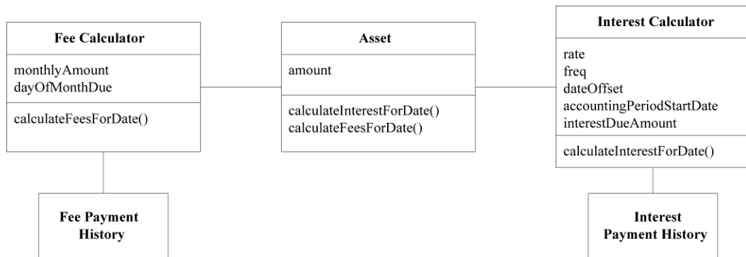
图9-4 笨拙的模型
