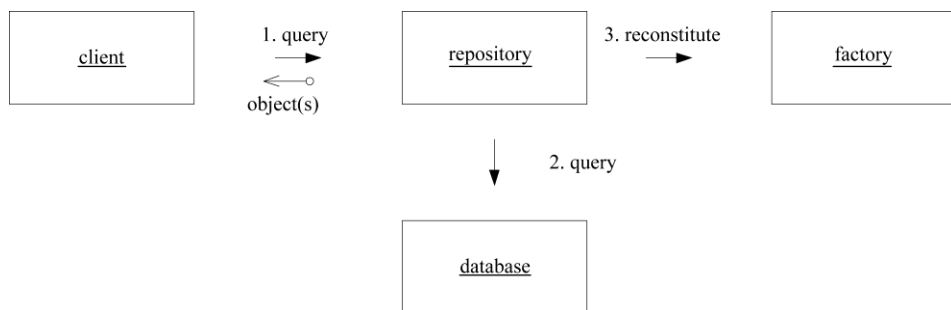
图6-22 REPOSITORY使用FACTORY来重建一个已有对象
