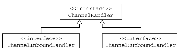
图 3-2 ChannelHandler 类的层次结构
