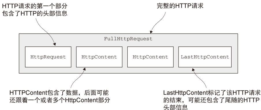
图 11-2 HTTP 请求的组成部分
