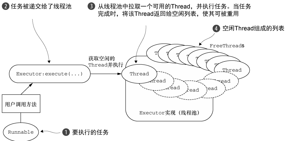
图 7-1 Executor 的执行逻辑
