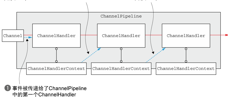
图 6-5 通过 Channel 或者 ChannelPipeline 进行的事件传播
