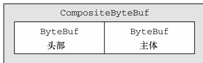
图 5-2 持有一个头部和主体的 CompositeByteBuffer
