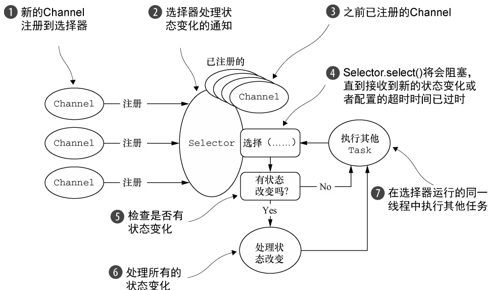
图 4-2 选择并处理状态的变化
