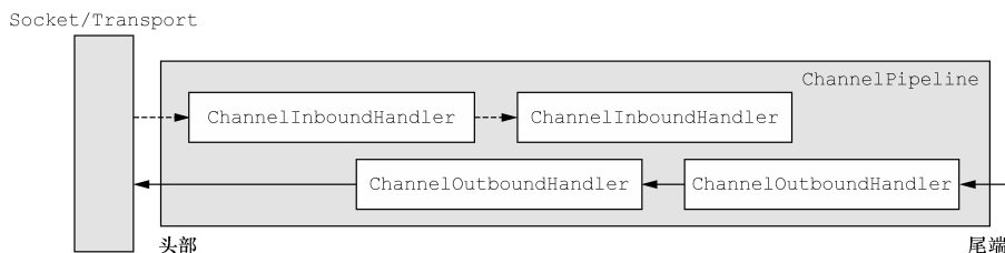
图 3-3 包含入站和出站 ChannelHandler 的 ChannelPipeline
