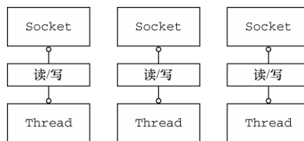
图 1-1 使用阻塞 I/O 处理多个连接
