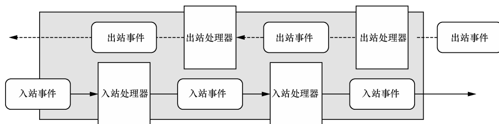
图 1-3 流经 ChannelHandler 链的进站事件和出站事件
