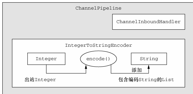
图 10-4 IntegerToStringEncoder
