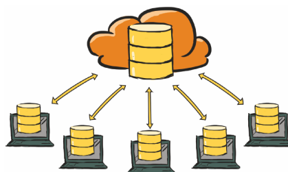
图 14-3 Firebase 的架构
