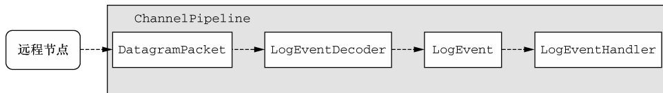
图 13-4 LogEventMonitor
