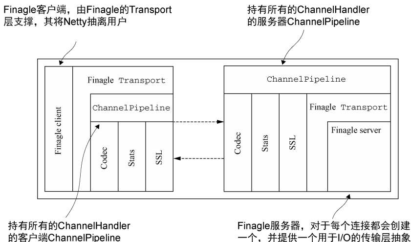
图 15-6 Netty 的使用
