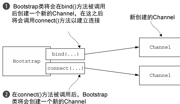
图 8-2 引导过程
