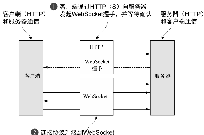
图 11-4 WebSocket 协议
