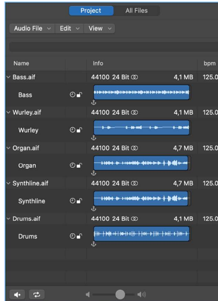
Project Browser
