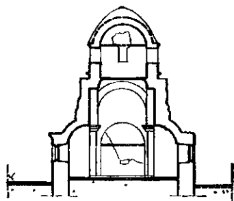
Ск. 22 — Попречни пресјек
