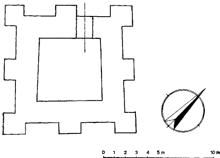
Ск. 12 — Тојаона, основица пирга
