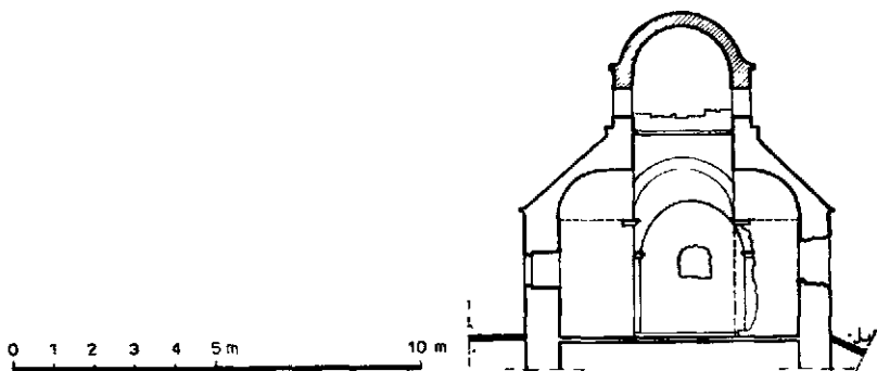
Ск. 18 — Попречни пресјек
