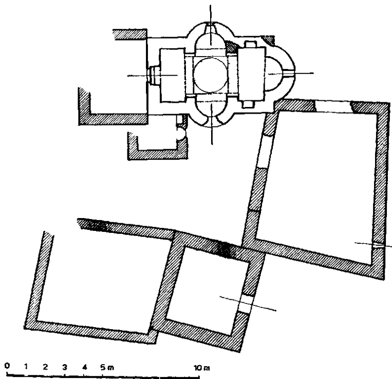
Ск. 20 — Морачник, Богородичин манастир, основица
