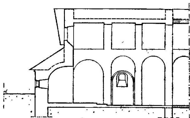
Ск. 26 — Подужни пресјек
