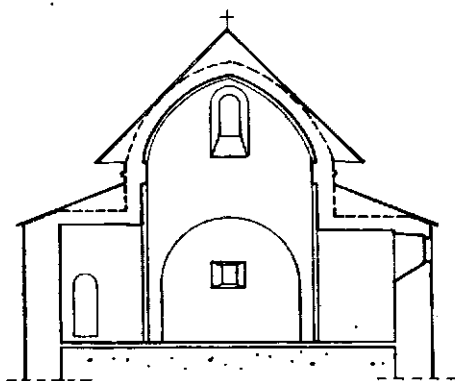
Ск. 28 — Попречни пресјек
