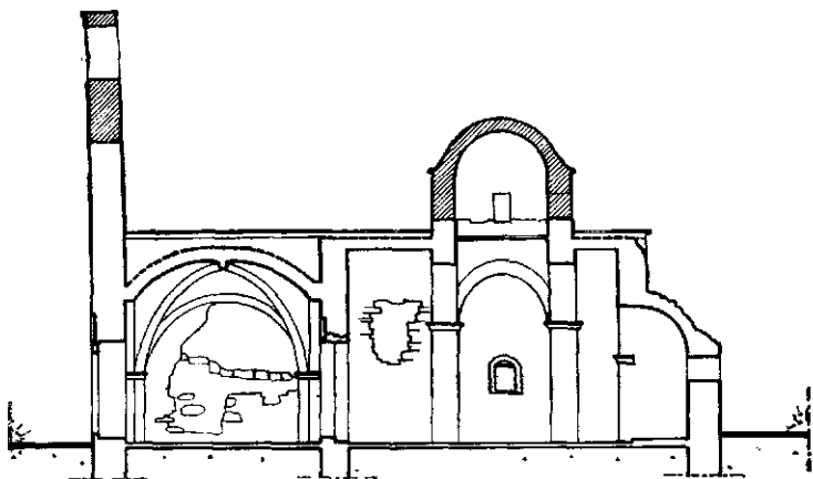
Ск. 16 — Подужни пресјек
