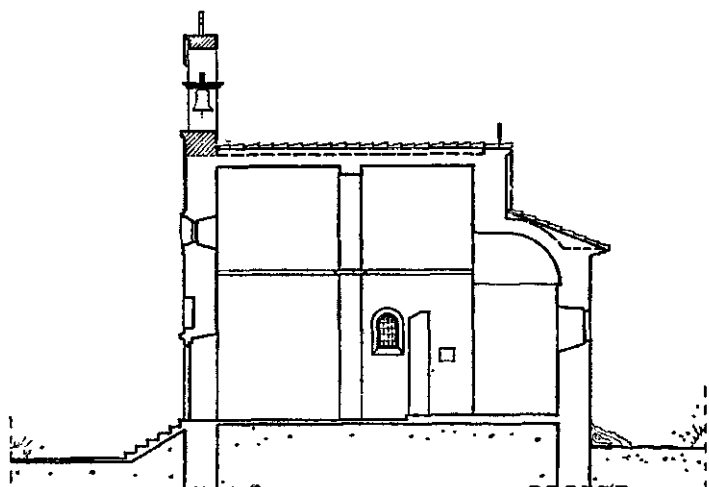
Ск. 32 — Подужни пресјек
