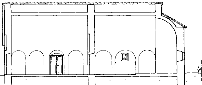
Ск. 23 — Подужни пресјек, реконструкција
