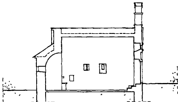
Ск. 35 — Подужни пресјек
