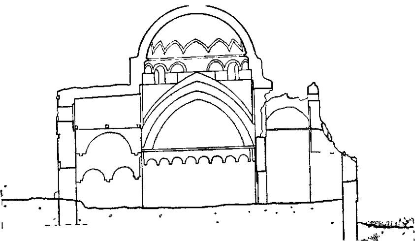
Ск. 30 Подужни пресјек
