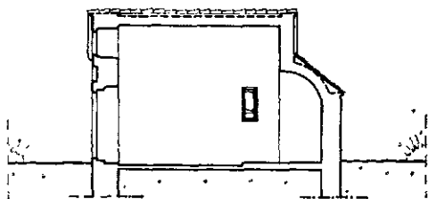
Ск. 51 — Подужни пресјек
