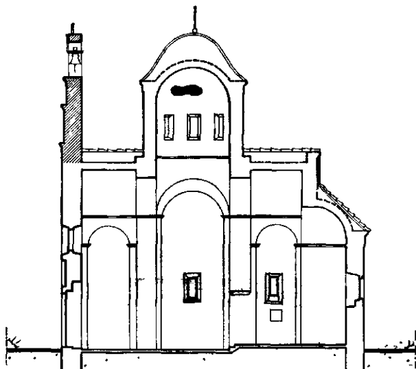
Ск. 38 — Подужни пресјек
