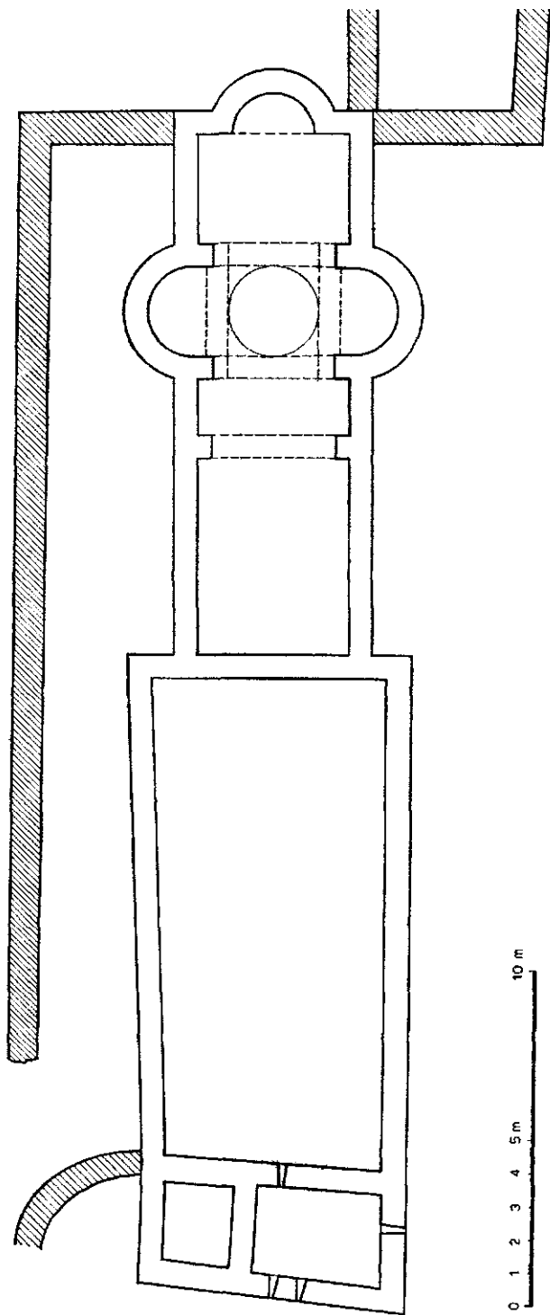
Ск. 19 — Црква Богородице Крајинске, основница
