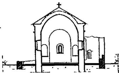
Ск. 50 — Попречни пресјек
