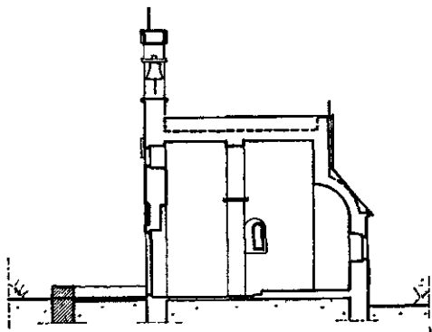
Ск. 48 — Подужни пресјек
