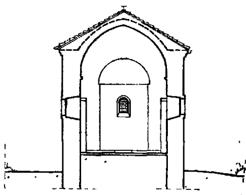
Ск. 34 — Попречни пресјек
