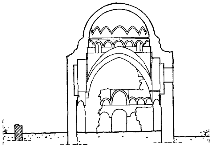
Ск. 29 — Попречни пресјек
