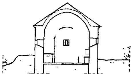
Ск. 37 — Попречни пресјек
