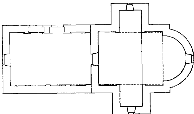
Ск. 24 — Реконструисана основица
