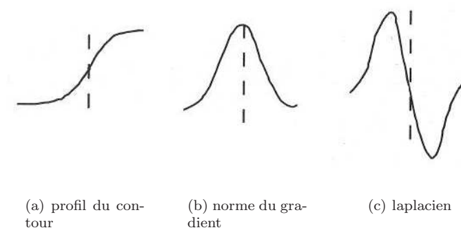
FIG. 5 – Opérateurs dérivatifs
