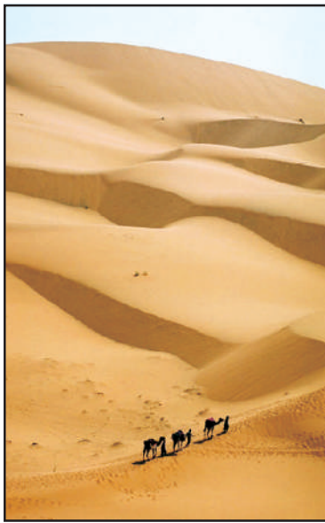
Fig. 3.9: Sand Dunes
