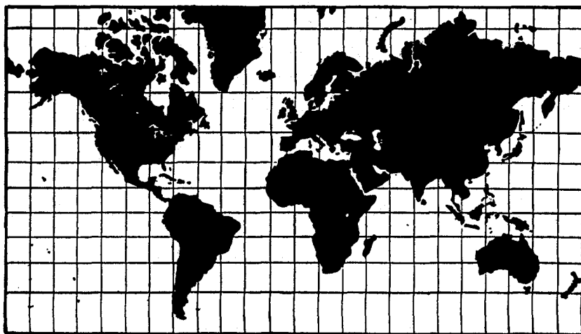
FIG. 67.—Mercator projection, from latitude 60^{\circ} south, to latitude 78^{\circ} north.
