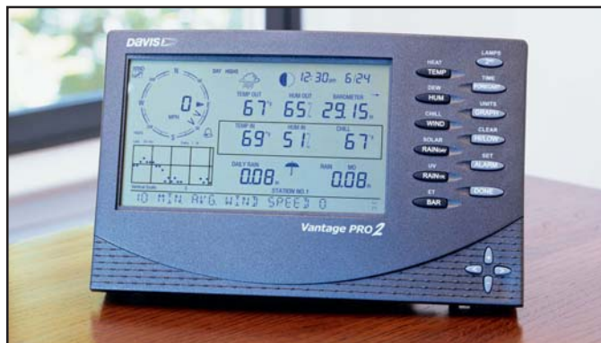
Vantage Pro2 Console
