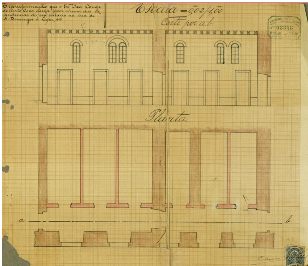
Figura 2 Planta referente a uma intervenção realizada em 1907, por um dos últimos descendentes do barão de Porto Covo. AML, Processo de obra n.º 4525 , processo n.º 3243/1.º REP/PG/1907, f. 2.
