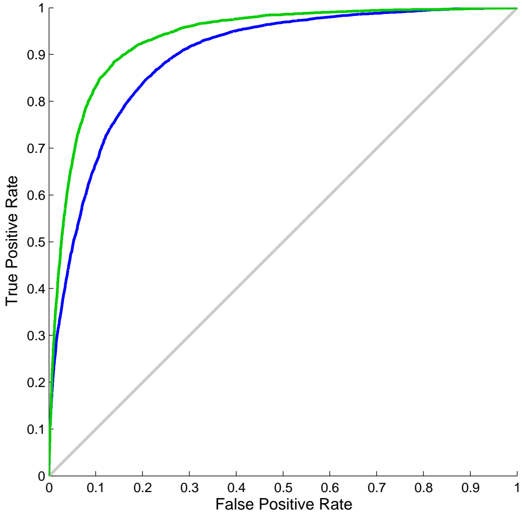
ROC
