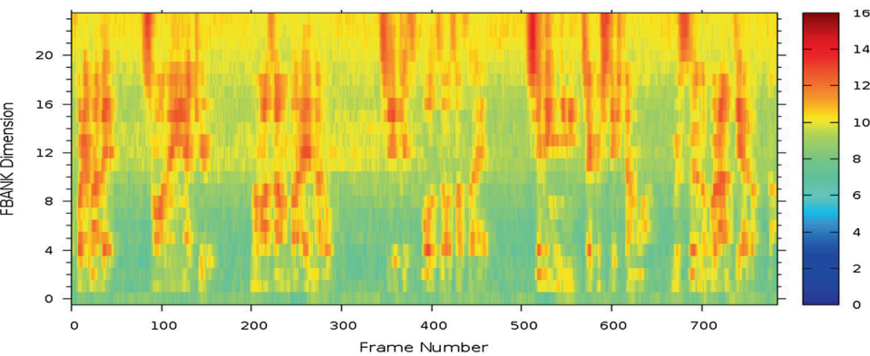
(D) Denormalized dereverberated feature vectors, \hat{S}(t) .
