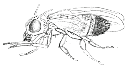
D. melanogaster
