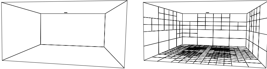
FIG. 1.5: Exemple de scène discrétisée. Une scène constituée de 6 polygones (à gauche) a été discrétisée en 525 surfaces élémentaires sur lesquelles la radiosité est approchée par une valeur uniforme.
