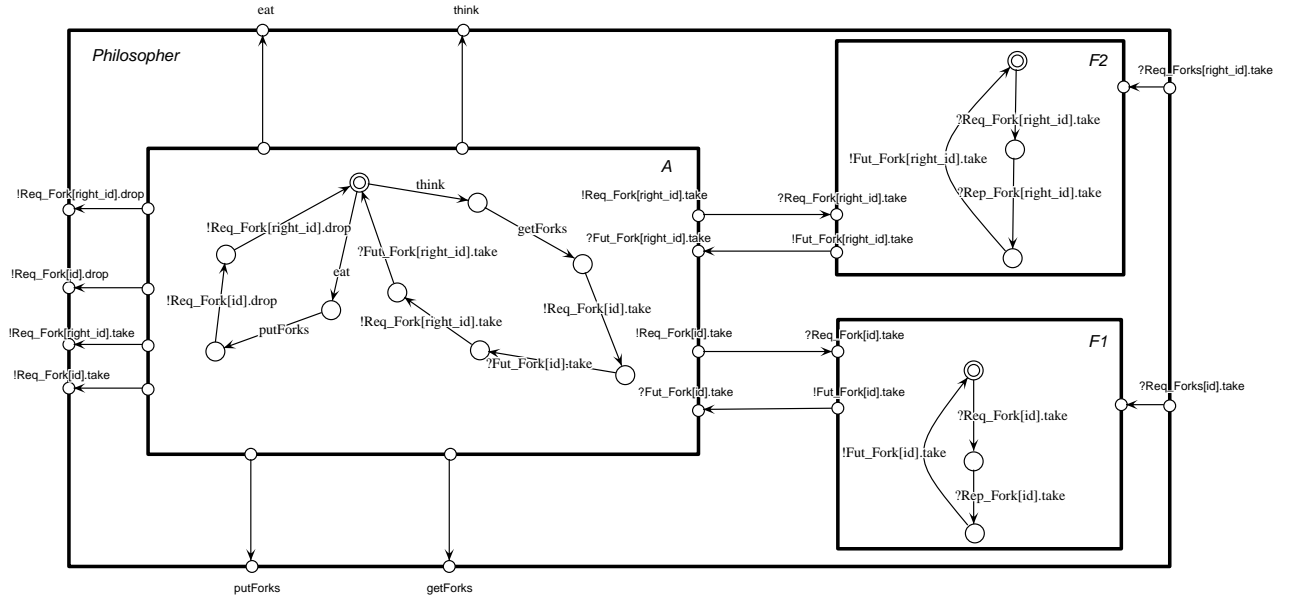
FIG. 3.12 – Comportement d'un Philosophe : LTSs des Futures et de runActivity
