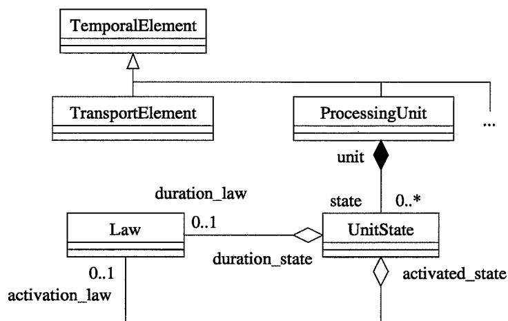
FIG. 9.7 – Extrait du métamodèle du sous-système opérationnel
