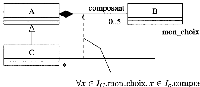
FIG. 9.9 – Extrait d'un métamodèle pour la vérification locale
