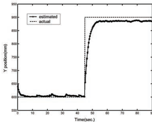
(b) Position estimation in y axis.
