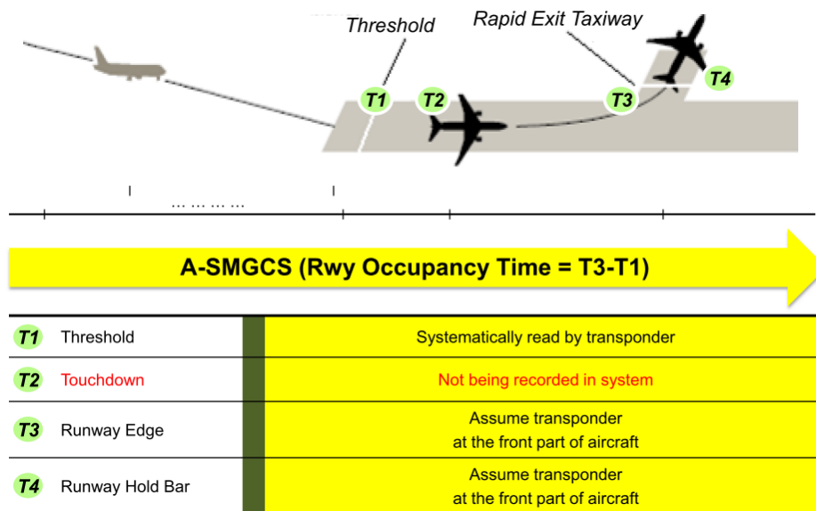
圖 19 ROTa Definition
