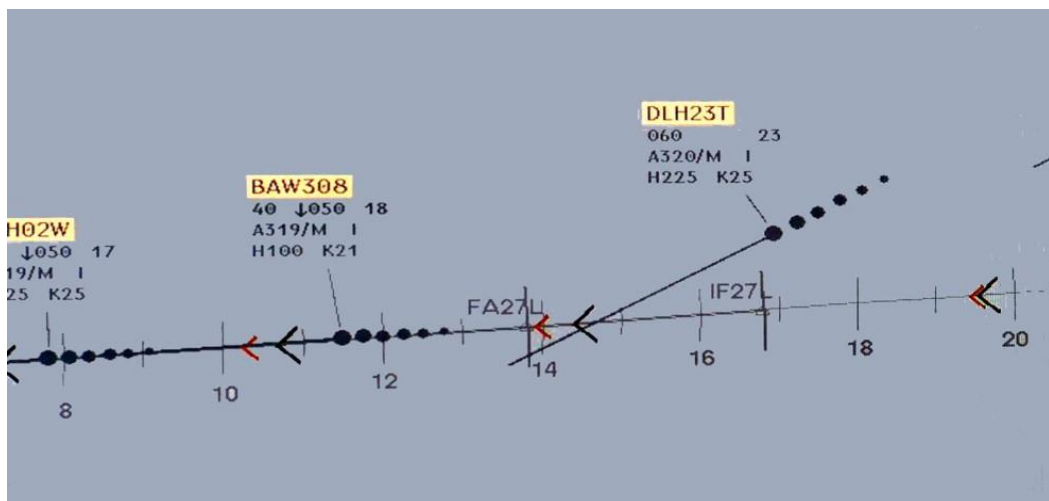
圖 10 TBS 的 HMI
