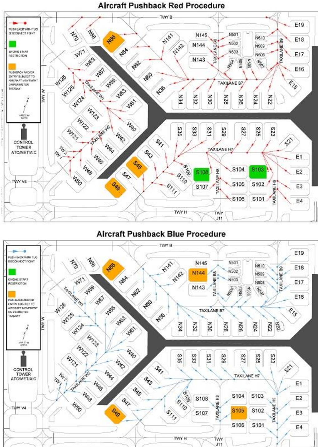
圖 17 Pushback Procedure
