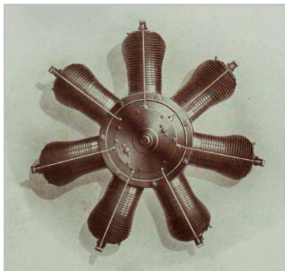
Gnome de 50 hp
