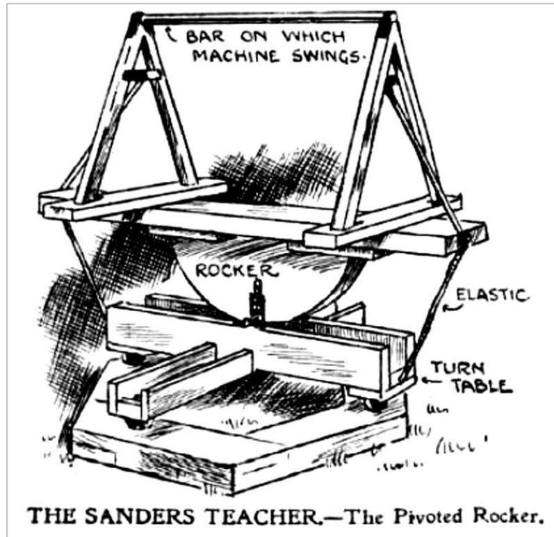
Detalle del sistema vasculante del simulador 20
