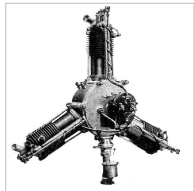
Anzani tipo Y de 35 hp
