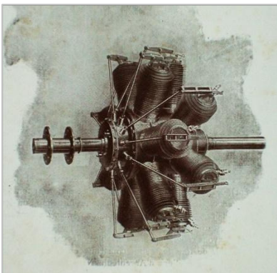
Gnome double Omega de 100 hp
