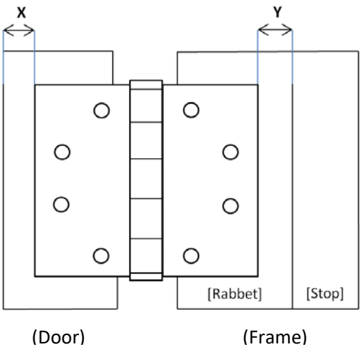
HINGE BACKSETS
