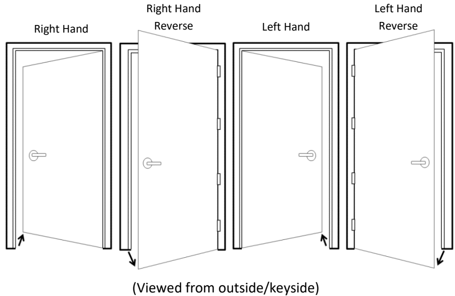
DOOR HANDING
