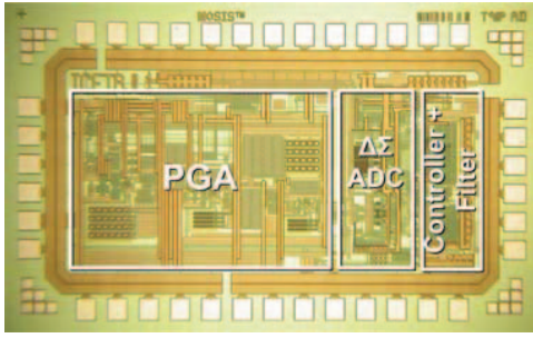
Fig. 5. Die Photo
