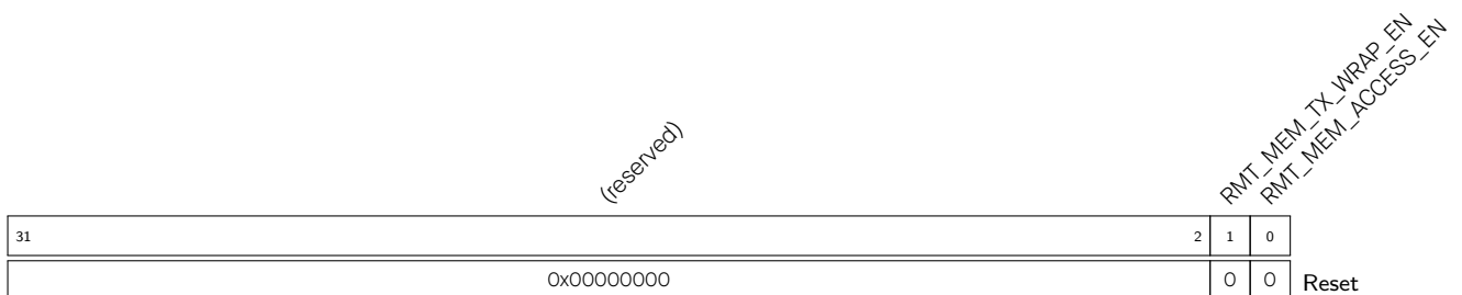
Register 15.9. RMT_APB_CONF_REG (0x00F0)
