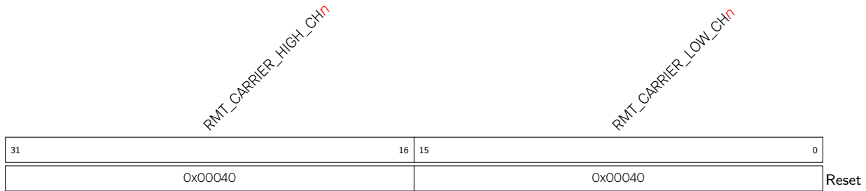
Register 15.7. RMT_CH n CARRIER_DUTY_REG ( n : 0-7) (0x00B0+4* n )
