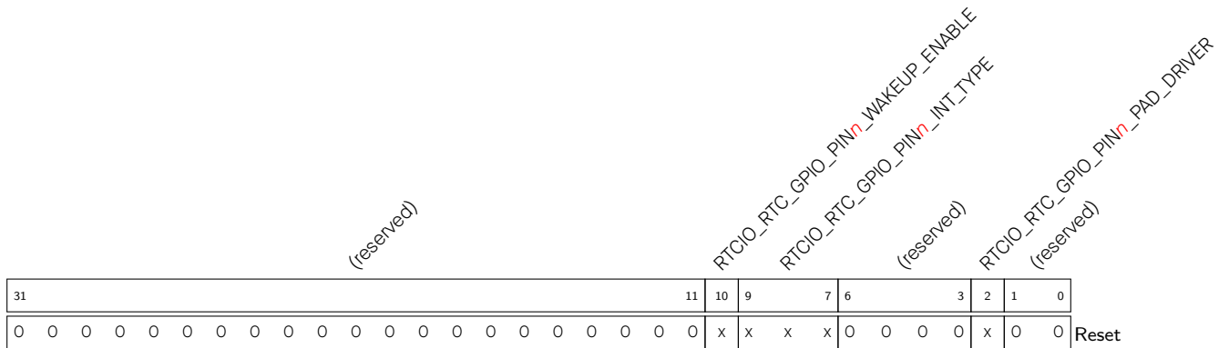
Register 4.45. RTCIO_RTC_GPIO_PIN n _REG ( n : 0-17) (0x28+4 \cdot n )
