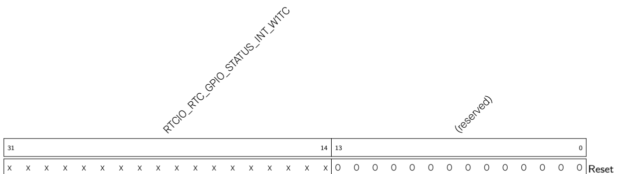
Register 4.43. RTCIO_RTC_GPIO_STATUS_W1TC_REG (0x0020)
