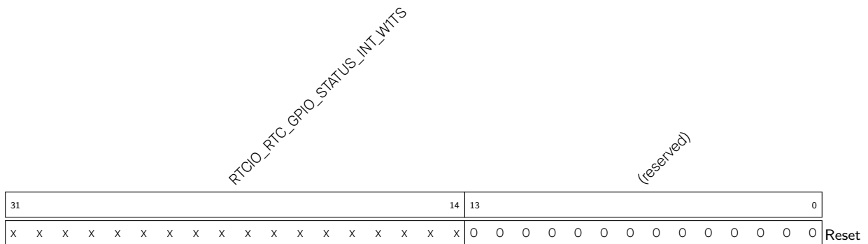
Register 4.42. RTCIO_RTC_GPIO_STATUS_W1TS_REG (0x001C)
