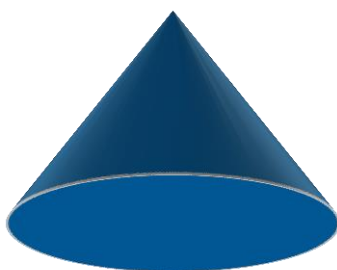
Cone
