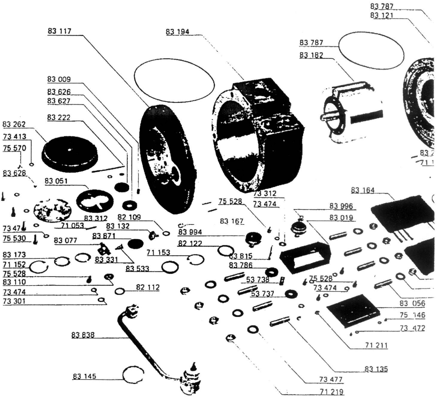
POMPE 2 100 PLANCHE 03
