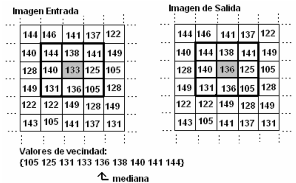
Figura 3. Funcionamiento filtrado de mediana.
