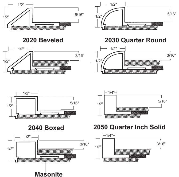
Premier Plus Frame Styles
