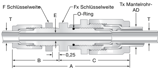
Mit Rohr dargestellt, O-Ring ist aus Aflas®.
